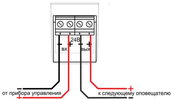
Рис. 2. Схема подключения оповещателя
