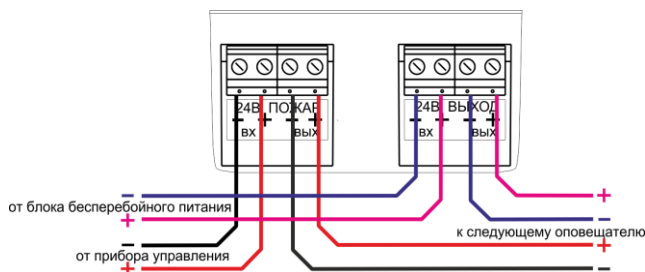
Рис.2 Схема подключения оповещателя
