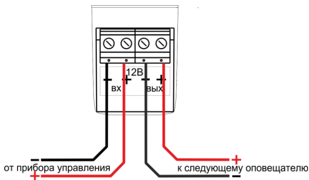
Рис. 2. Схема подключения оповещателя
