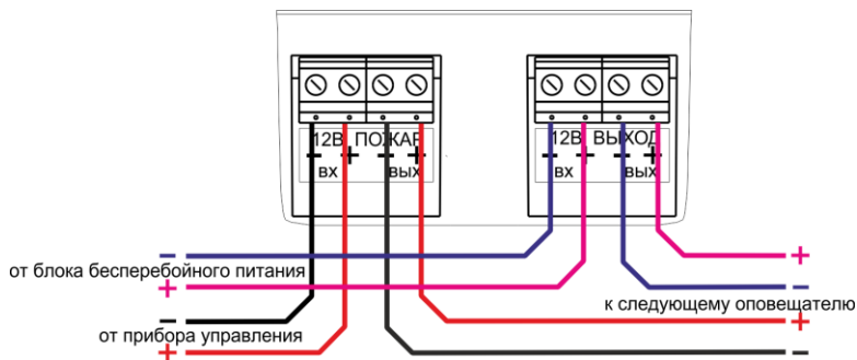
Рис. 2. Схема подключения оповещателя
