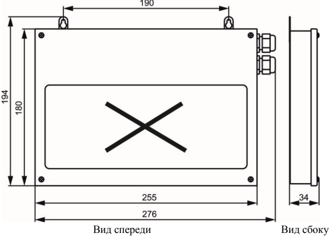
Рис. 1. Внешний вид, габаритные и установочные размеры корпуса оповещателя
