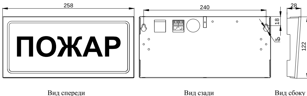
Рис. 1. Внешний вид, габаритные и установочные размеры корпуса оповещателя
