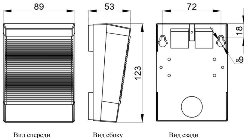
Рис. 1. Внешний вид, габаритные и установочные размеры корпуса оповещателя
