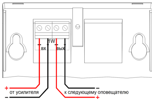
Рис. 2. Схема подключения оповещателя
