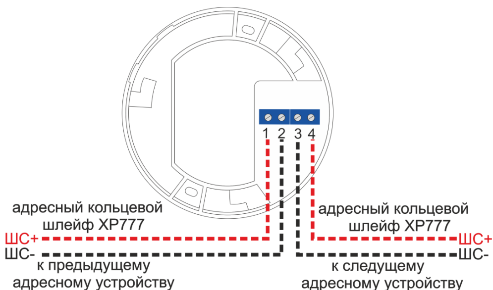
Рисунок 28. Схема подключения RF05-T
