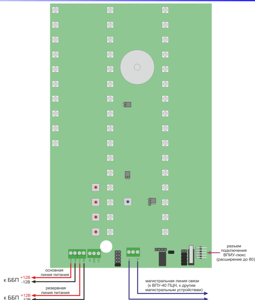
Рисунок 17. Схема подключения ВПИУ-люкс магистральная
