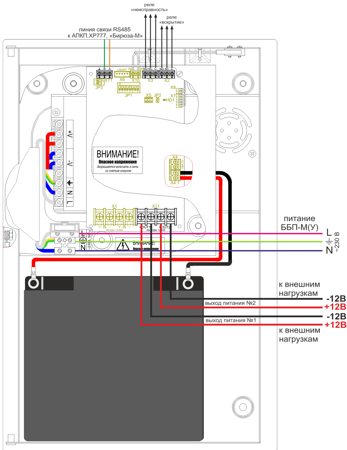
Рисунок 78. Схема подключения БПП-М-4/12(У), БПП-М-8/12(У), БПП-М-12/12(У)
