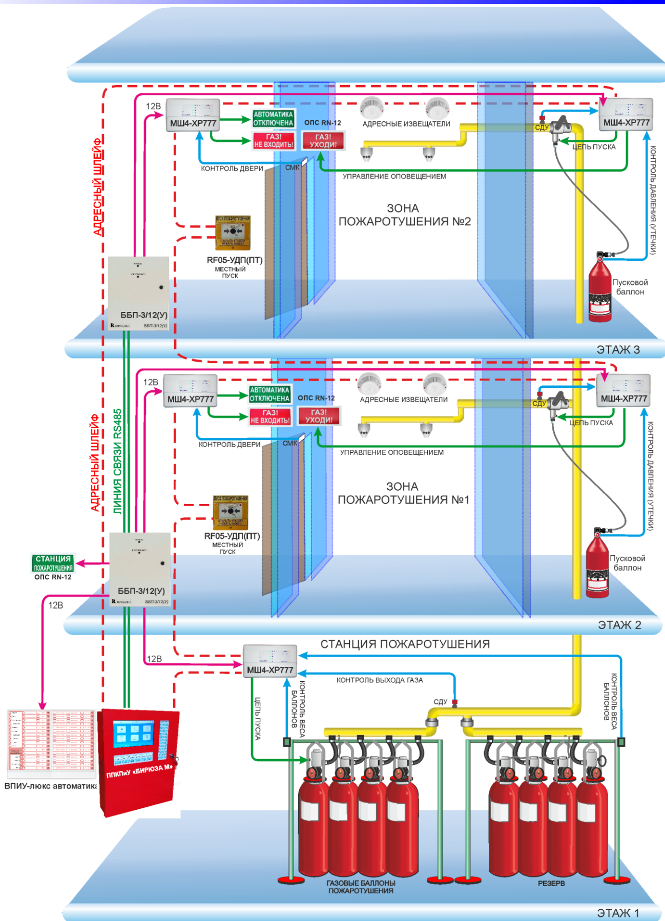
Рисунок 107. Автоматизация системы централизованного газового АПТ
