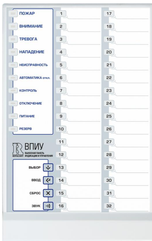
Рисунок 65. Внешний вид ВПИУ-люкс (базовая)
