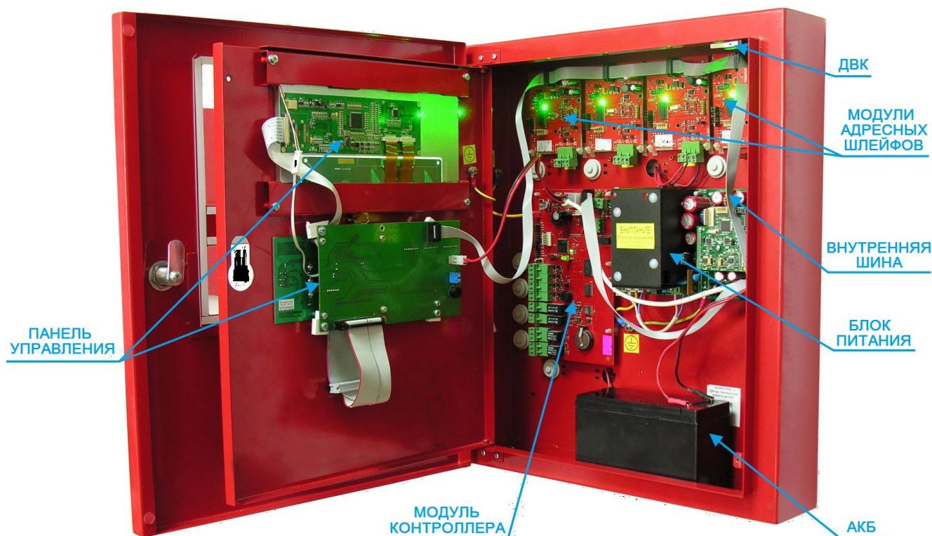
Рисунок 9. Внешний вид АПКП.ХРА6 и АПКП.ХР777 с открытой монтажной панелью.
