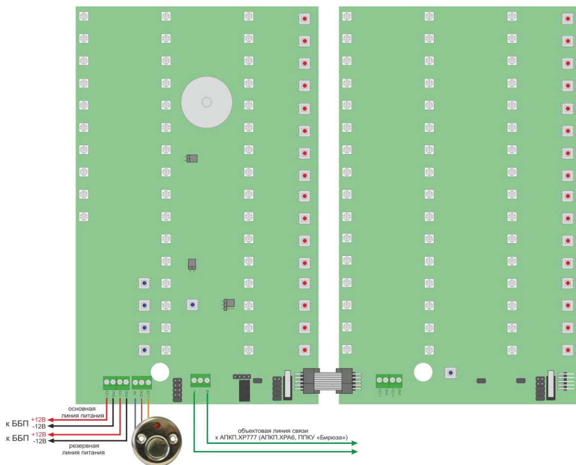
Рисунок 68. Схема подключения ВПИУ-люкс автоматика
