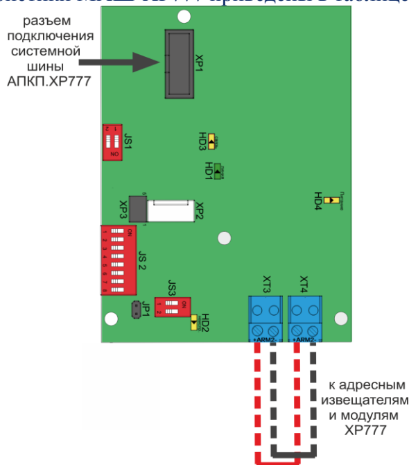
Рисунок 18. Схема подключения МАШ-ХР777
