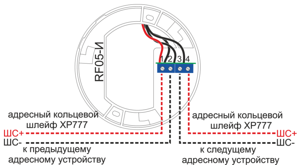
Рисунок 31. Схема подключения RF05-II
