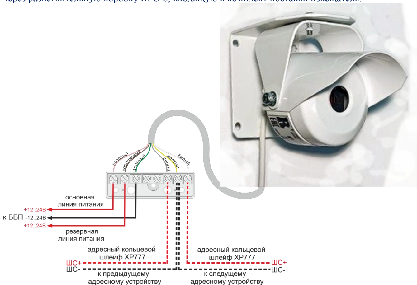
Рисунок 42. Внешний вид и схема подключения RF05-ИПП(01)
