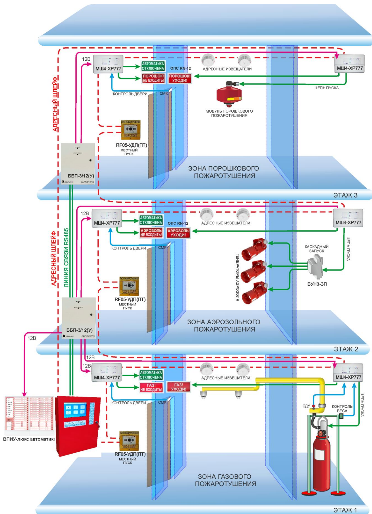
Рисунок 108. Автоматизация систем модульного пожаротушения
