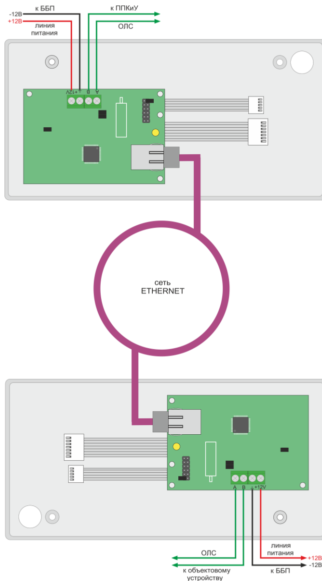
Рисунок 91. Схема подключения ИС-ЕТН/485 для организации связи ППКПиУ с ОУ
