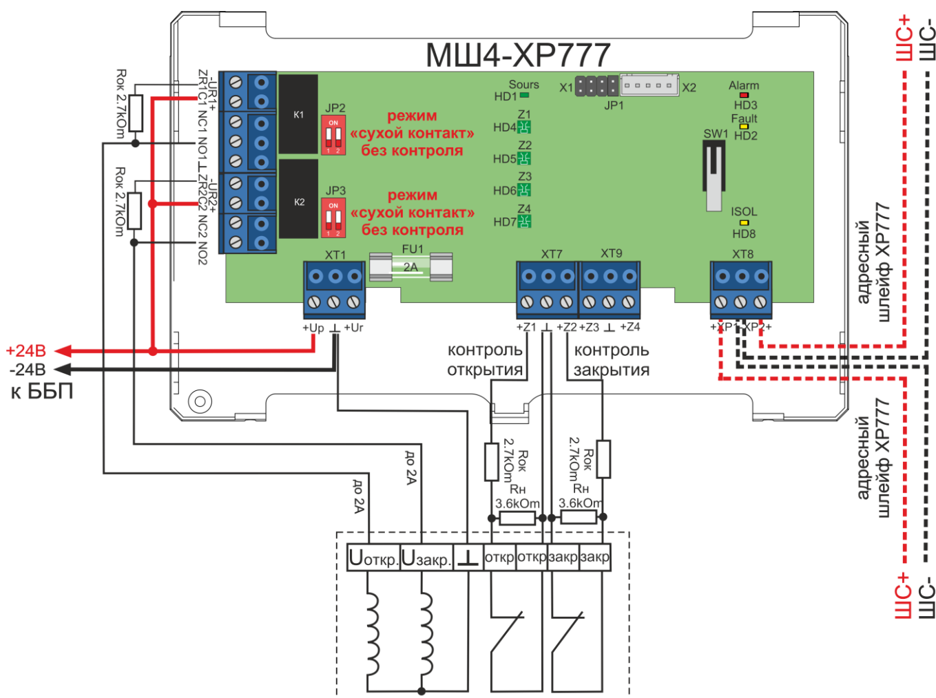
Рисунок 102. Схема подключения реверсивного 3-х проводного привода с напряжением питания 24В
