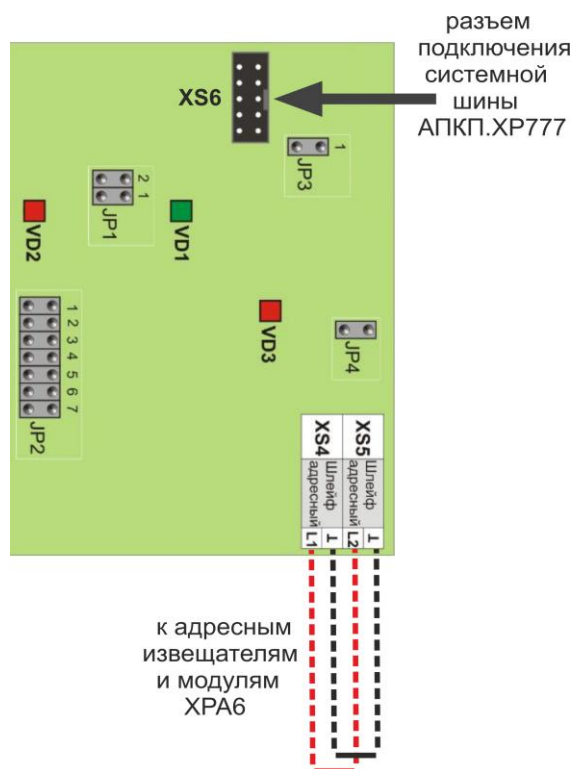
Рисунок 52. Схема подключения МАШ-ХРА6
