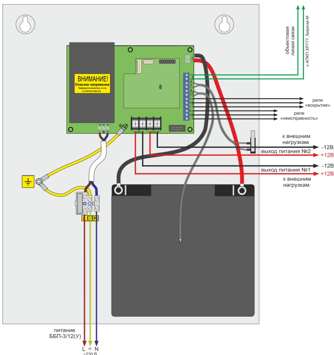
Рисунок 72. Схема подключения ББП-3/12(У)
