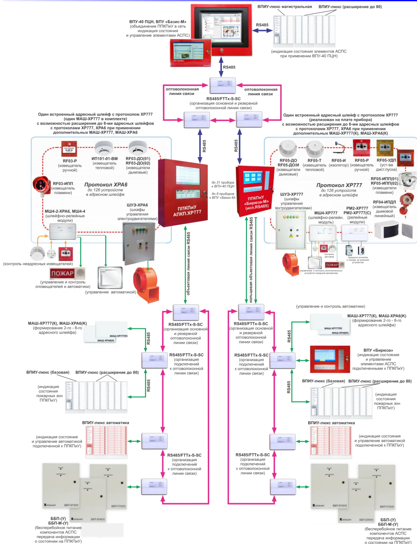
Рисунок 2. Структурная схема АСПС при использовании оптоволоконных линий связи
