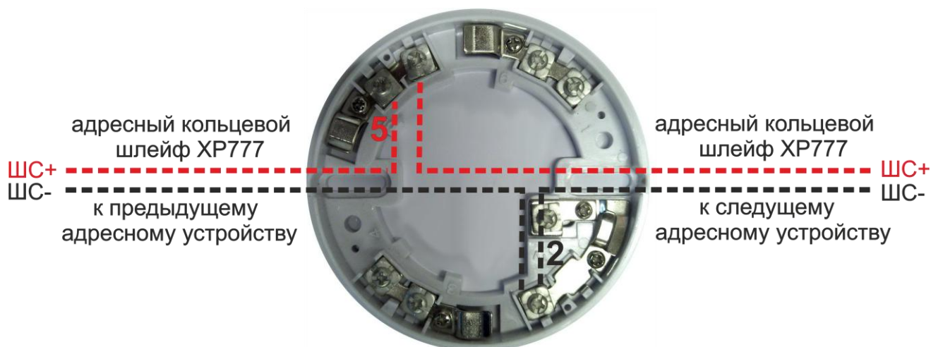
Рисунок 26. Схема подключения ИП101-02-ВМ
