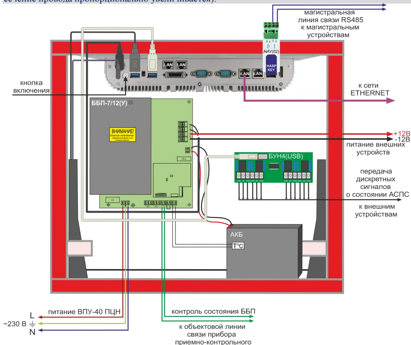
Рисунок 5. Структурная схема внутренних и внешних соединений ВПУ-40 ПЦН
