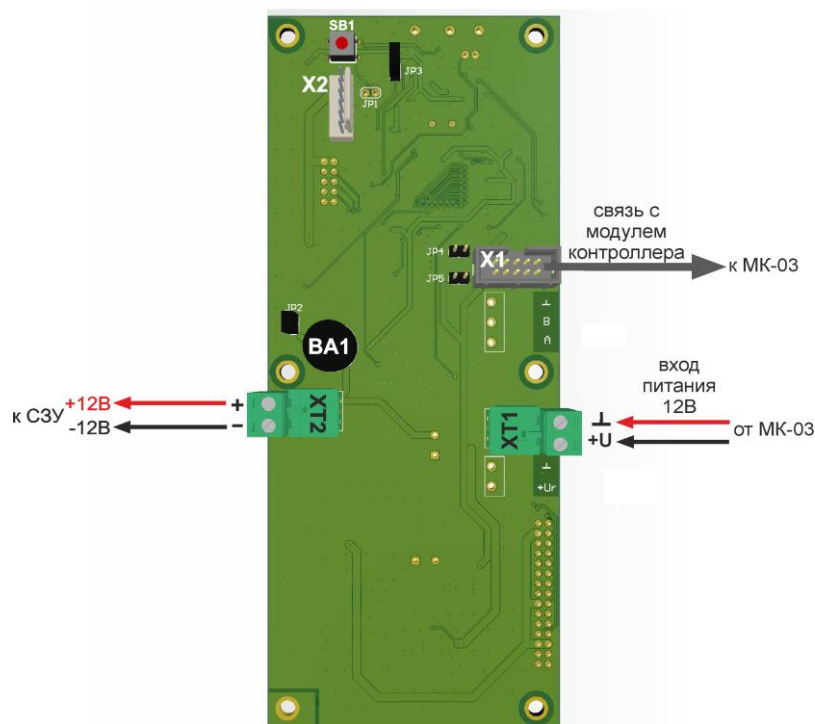
Рисунок 15. Внешний вид и схема подключения платы управления ПУ «Бирюза»
