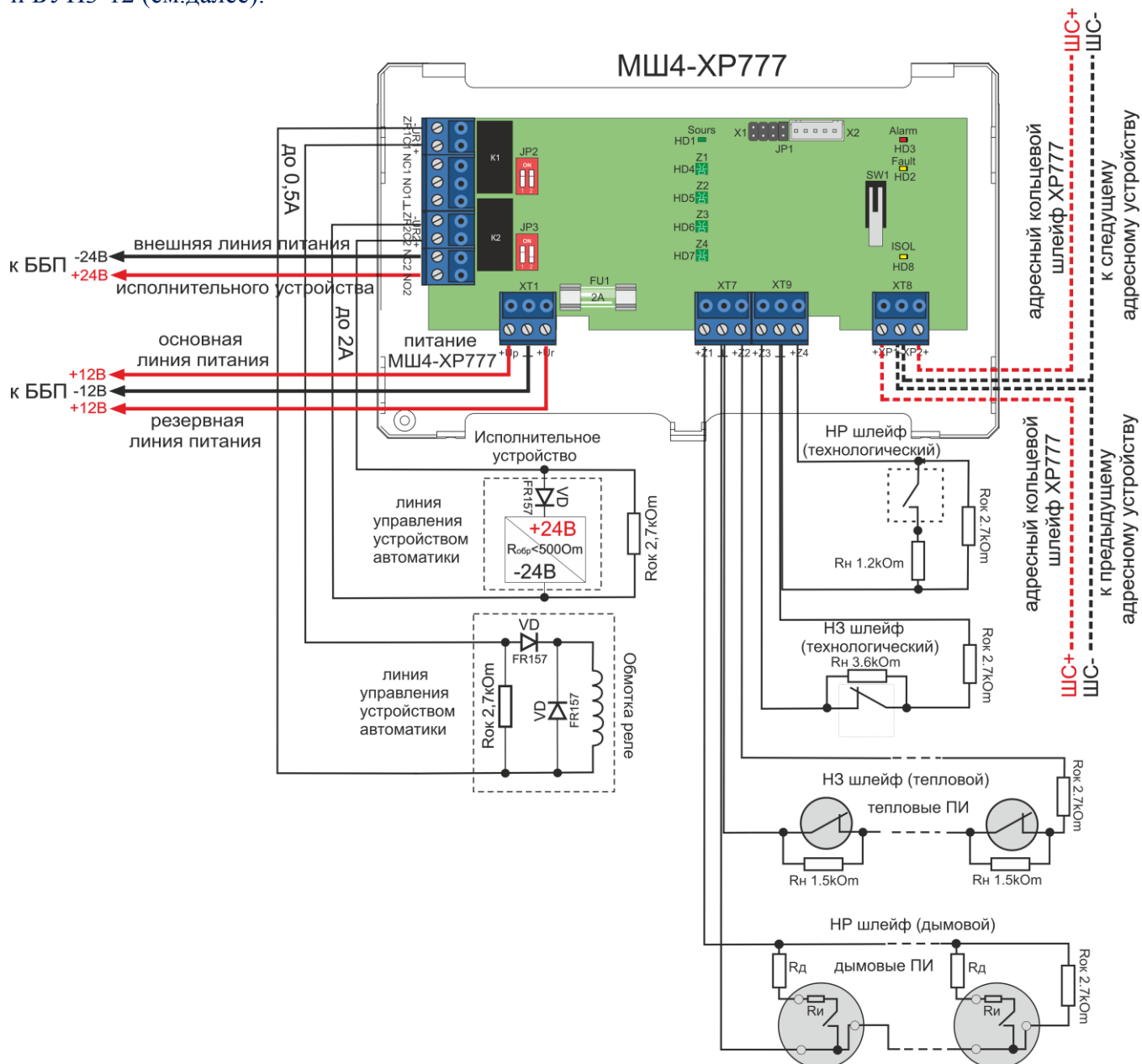
Рисунок 48. Схема подключения МШ4-ХР777
