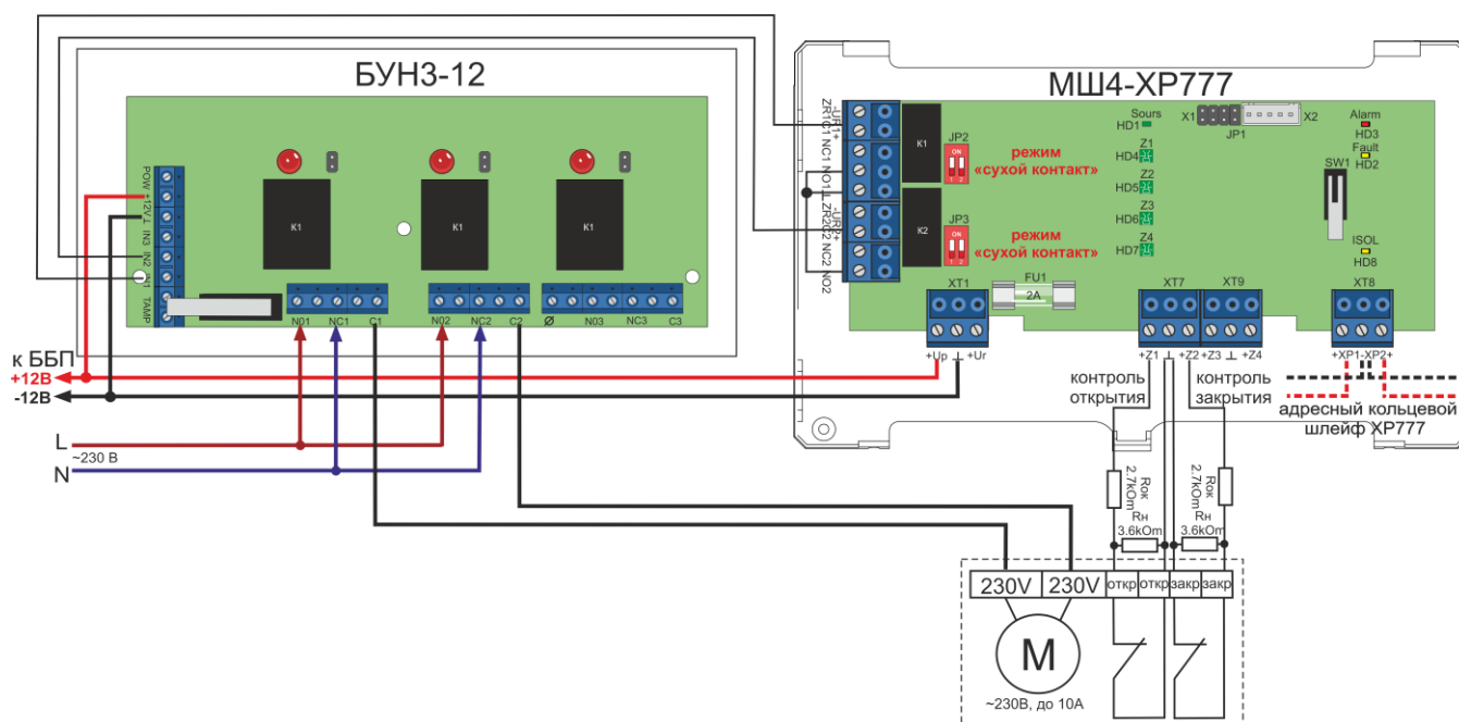
Рисунок 106. Схема подключения реверсивного 2-х проводного привода с напряжением питания 230В
