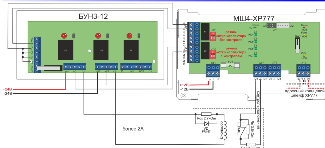
Рисунок 100. Схема подключения электромагнитного привода с напряжением питания 24В и током потребления свыше 2А
