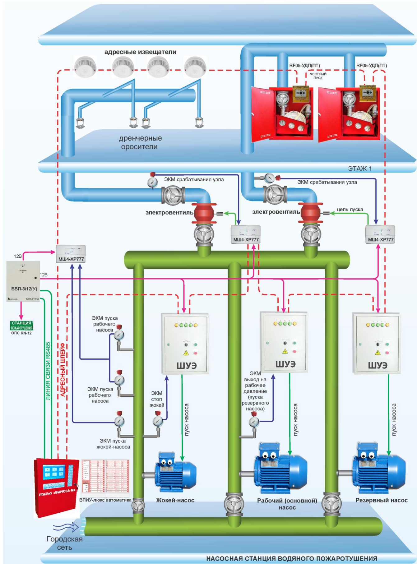
Рисунок 111. Автоматизация дренчерной установки системы водяного АПТ
