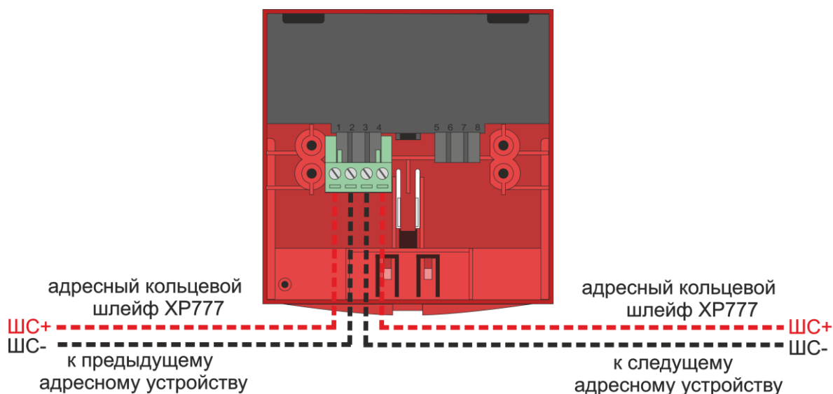
Рисунок 34. Схема подключения RF04-P
