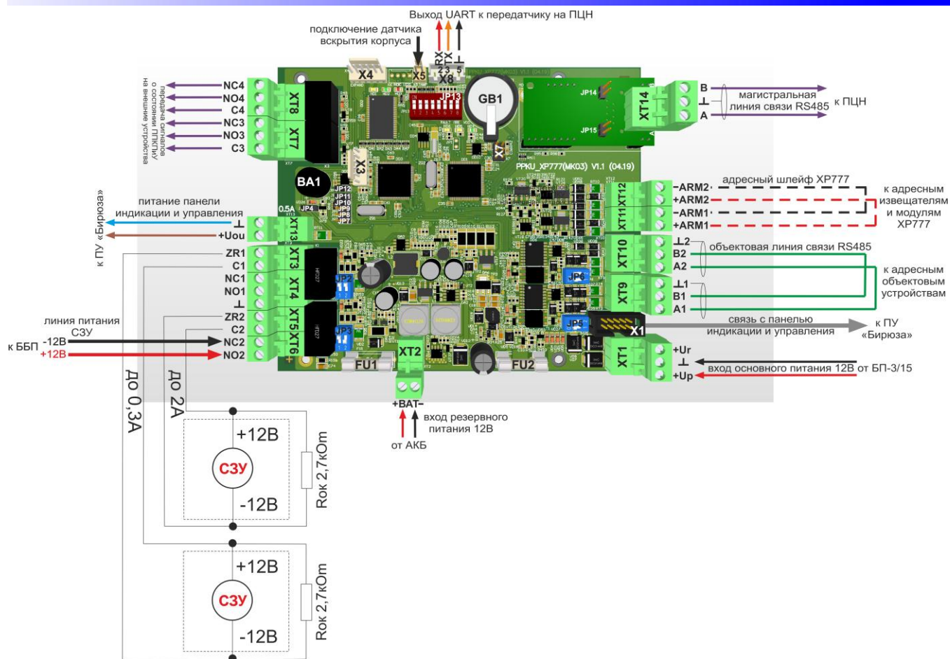
Рисунок 13. Схема подключения МК-03 ППКПиУ «Бирюза-М» (исп. RS485)
