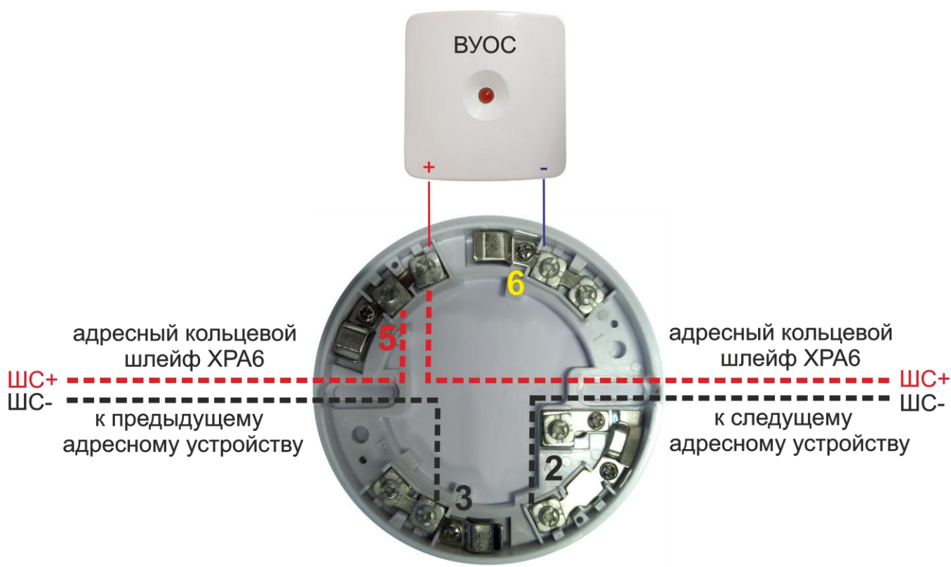
Рисунок 55. Схема подключения RF03-ДО(01) и RF03-ДО(02)
