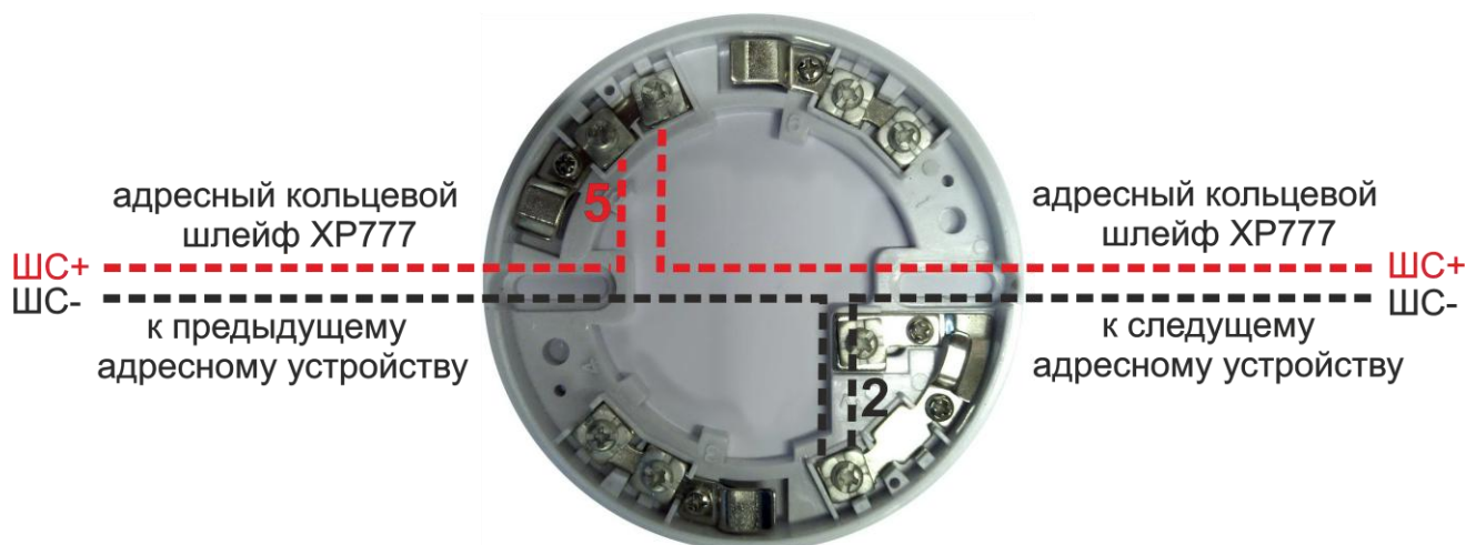
Рисунок 21. Схема подключения RF04-ДО
