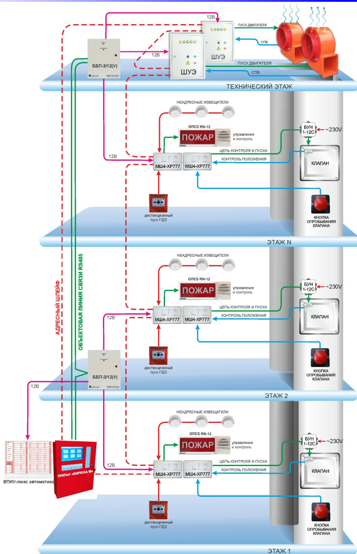
Рисунок 97. Построение системы ПДЗ с использованием неадресных извещателей
