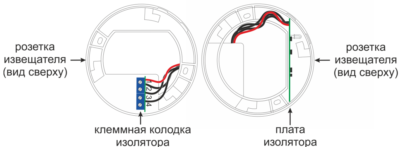
Рисунок 30. Установка RF05-II в розетку извещателя
