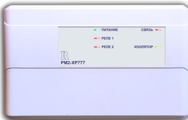
Рисунок 49. Внешний вид PM2-XP777 и PM2-XP777(C)
