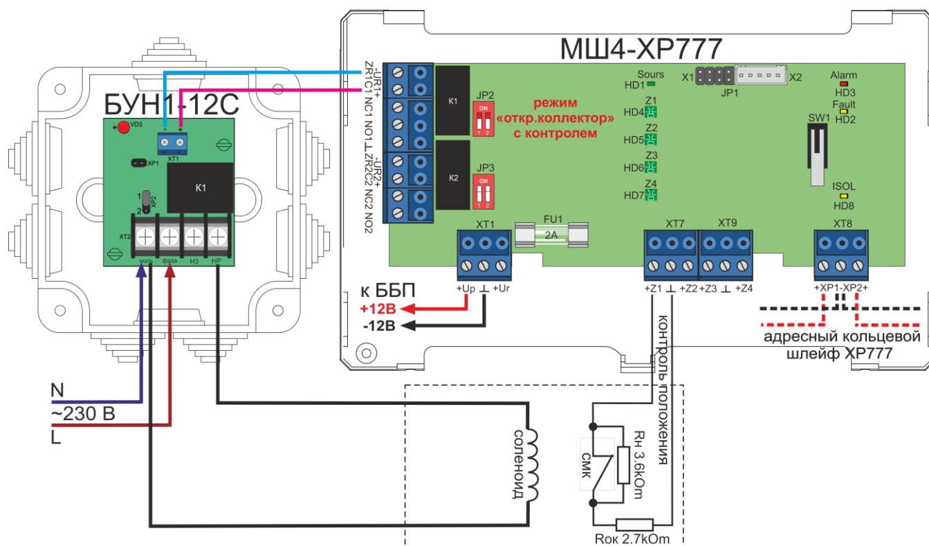
Рисунок 101. Схема подключения электромагнитного привода с напряжением питания 230В
