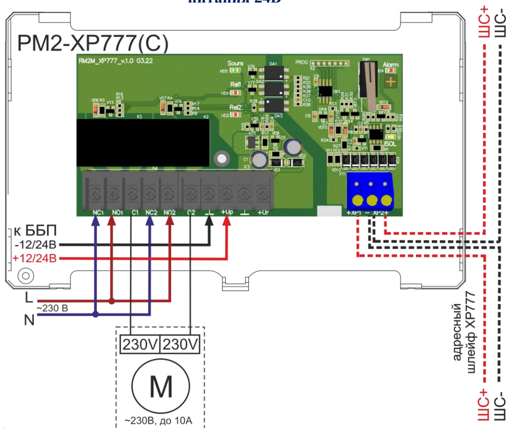
Рисунок 105. Схема управления 2-х проводным реверсивным приводом с напряжением питания 230В
