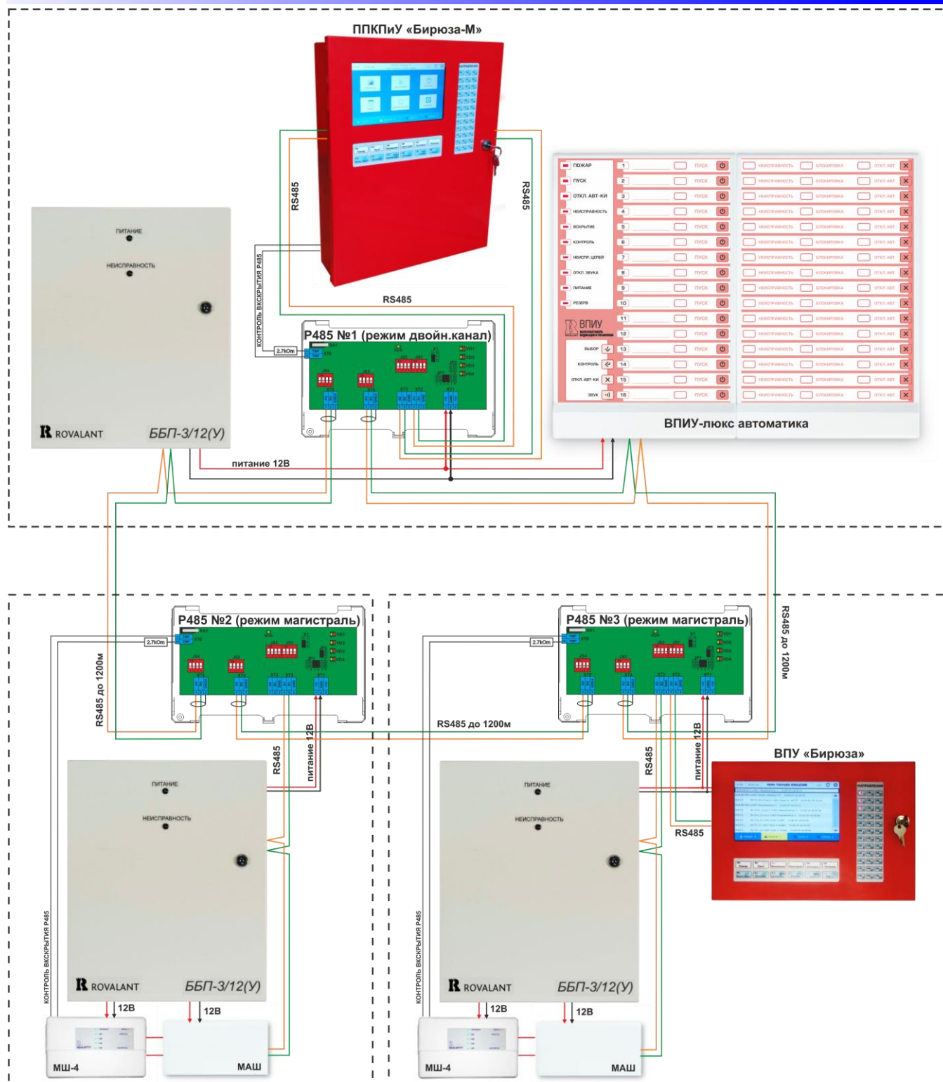
Рисунок 86. Схема организации защищенной ОЛС для ППКПиУ «Бирюза-М»
