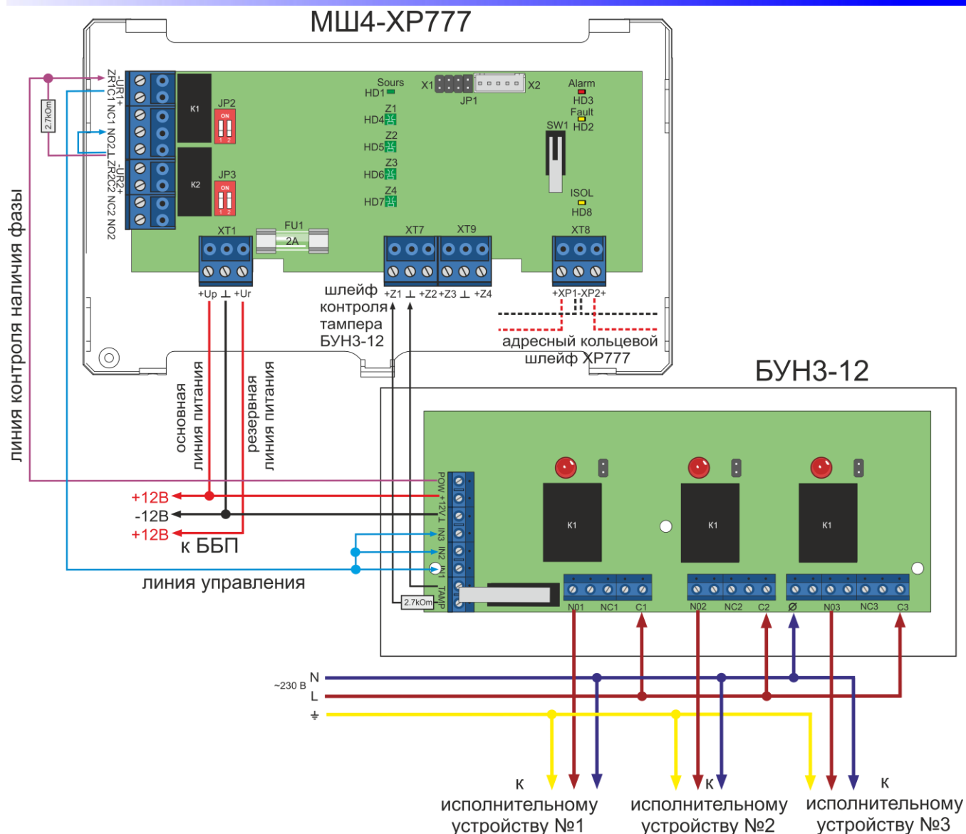
Рисунок 94. Схема подключения БУНЗ-12 к МШ4-ХР777
