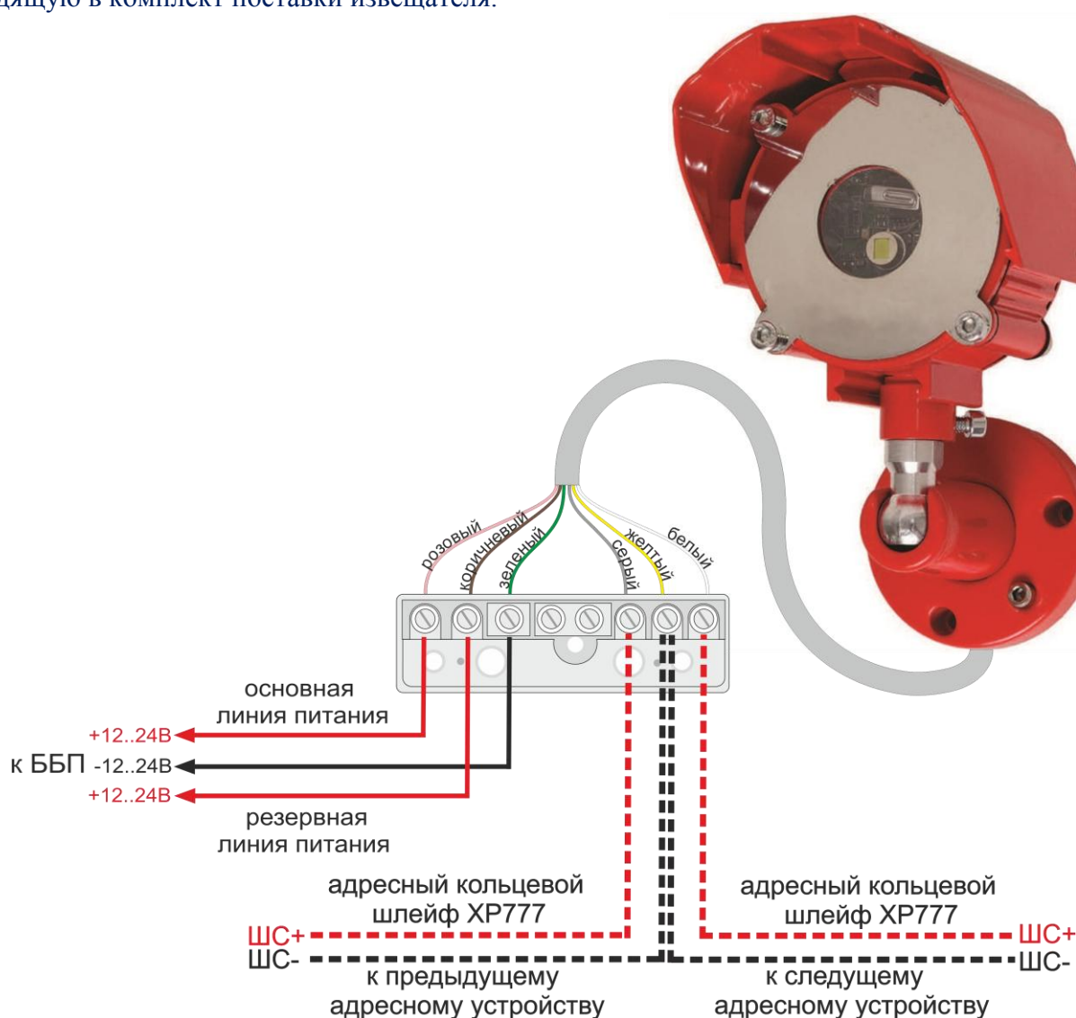
Рисунок 43. Внешний вид и схема подключения RF05-ИПП(02)
