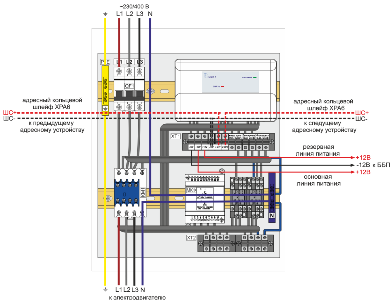
Рисунок 62. Схема подключения ШУЭ-ХРА6
