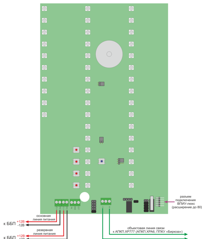
Рисунок 66. Схема подключения ВПИУ-люкс (базовая)
