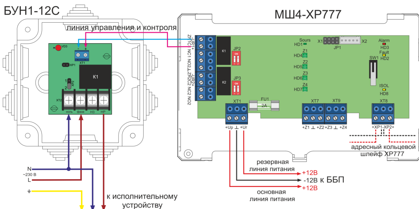
Рисунок 92. Схема подключения БУН1-12С к МШ4-ХР777
