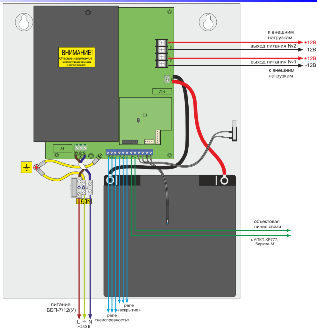
Рисунок 74. Схема подключения БП-7/12(У)
