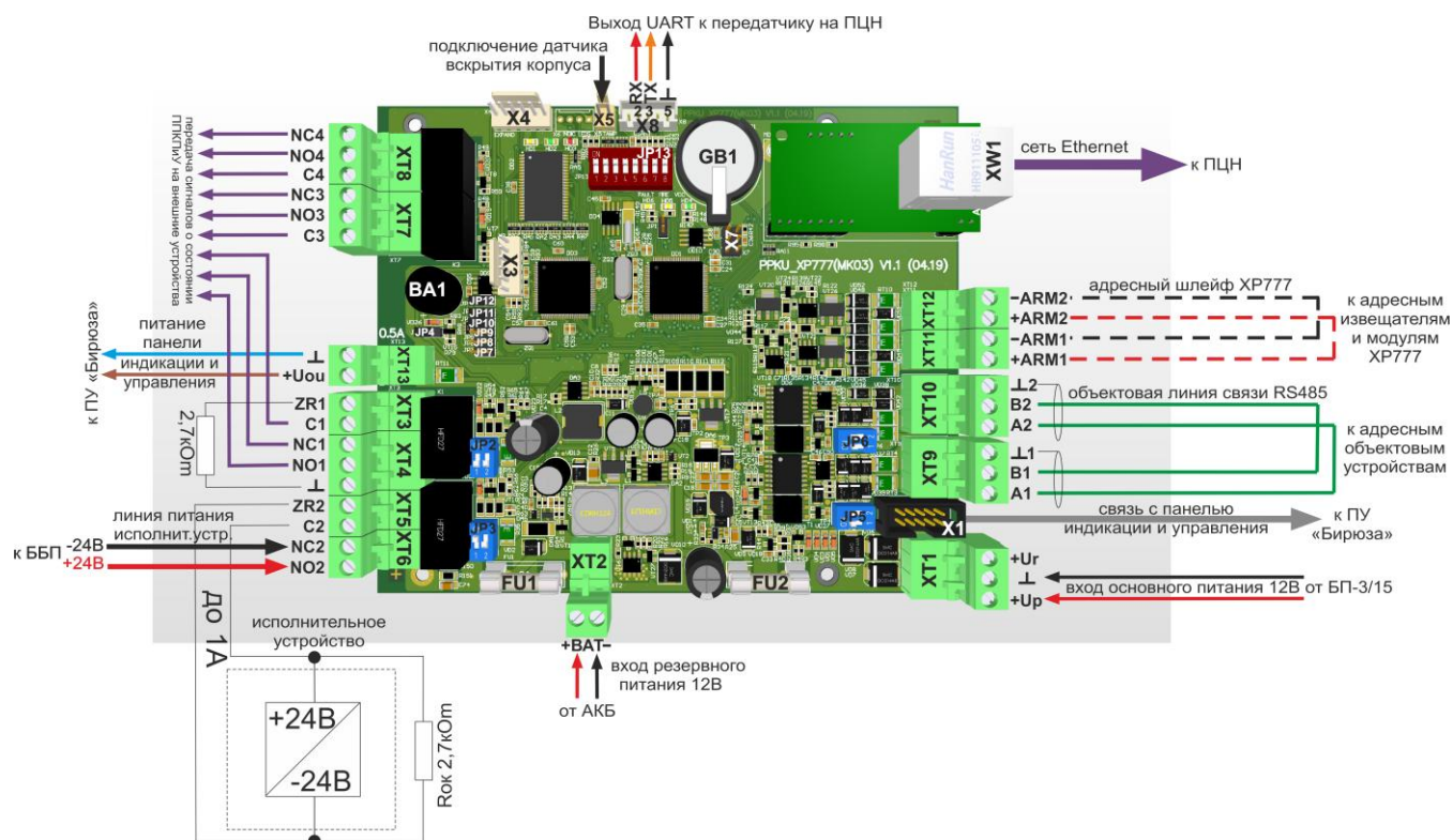
Рисунок 14. Схема подключения МК-03 ППКПиУ «Бирюза-М» (исп. Ethernet)
