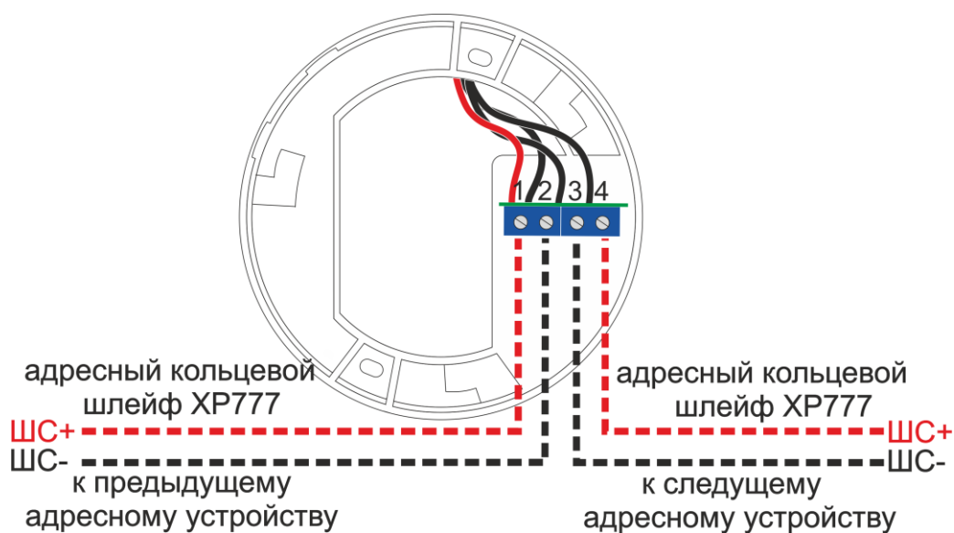
Рисунок 24. Схема подключения RF05-ДО/И
