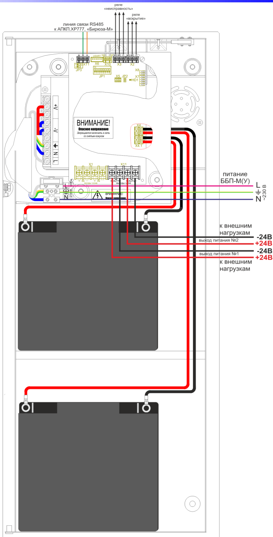
Рисунок 80. Схема подключения БП-М-4/24(У), БП-М-6/24(У), БП-М-8/24(У)
