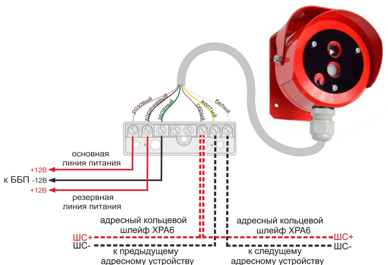
Рисунок 60. Внешний вид и схема подключения RF03-ИПП
