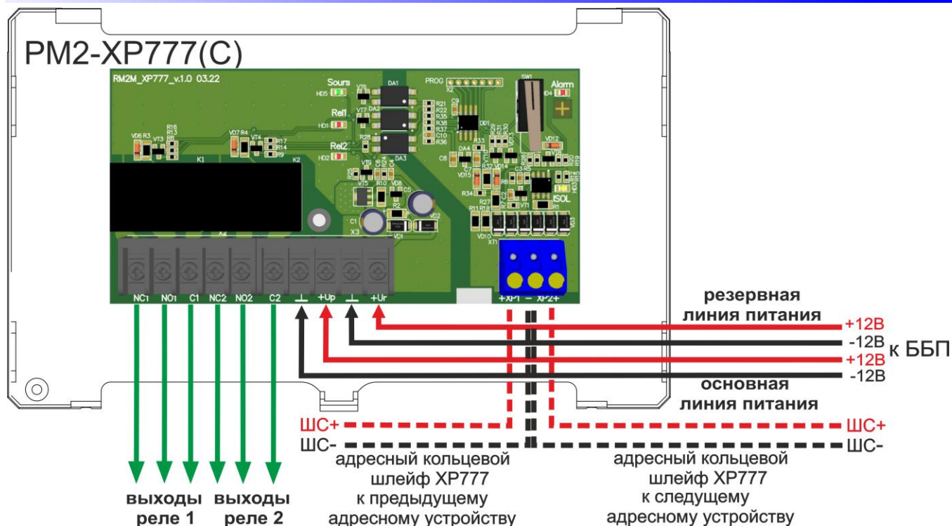
Рисунок 51. Внешний вид платы и схема подключения PM2-XP777(C)
