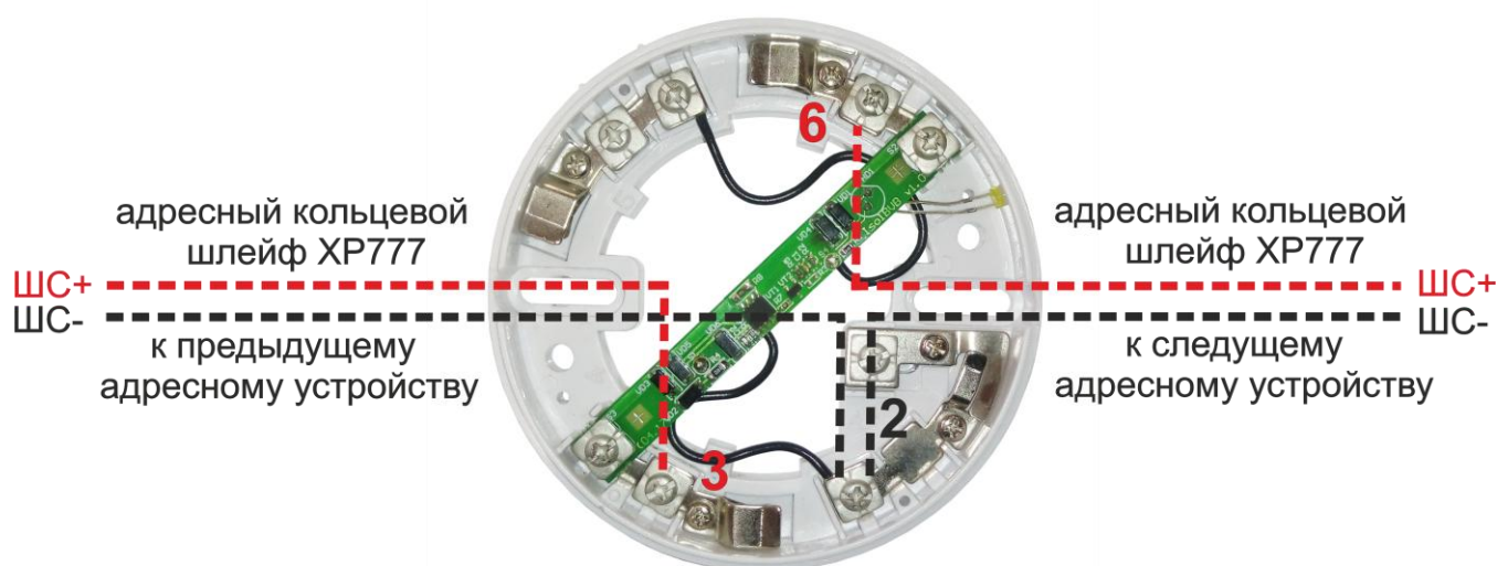
Рисунок 29. Внешний вид и схема подключения изолирующего основания XR777
