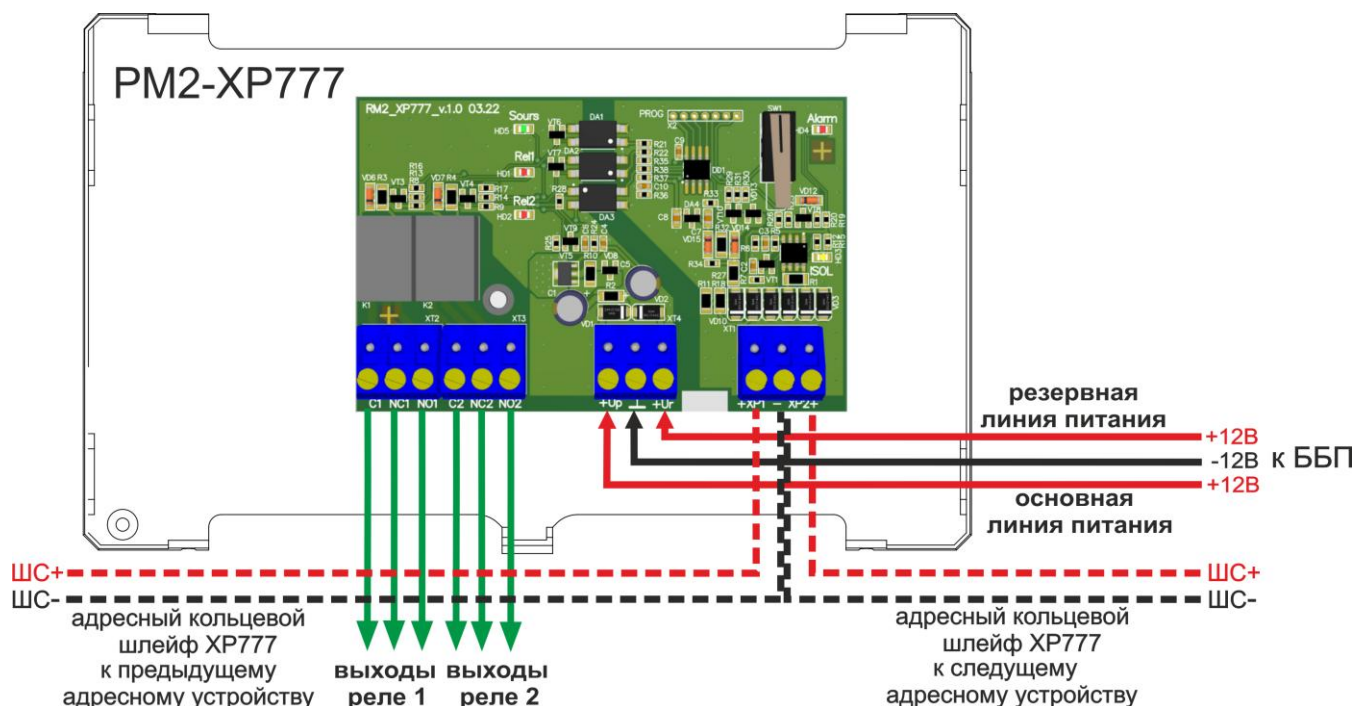
Рисунок 50. Внешний вид платы и схема подключения PM2-XP777
