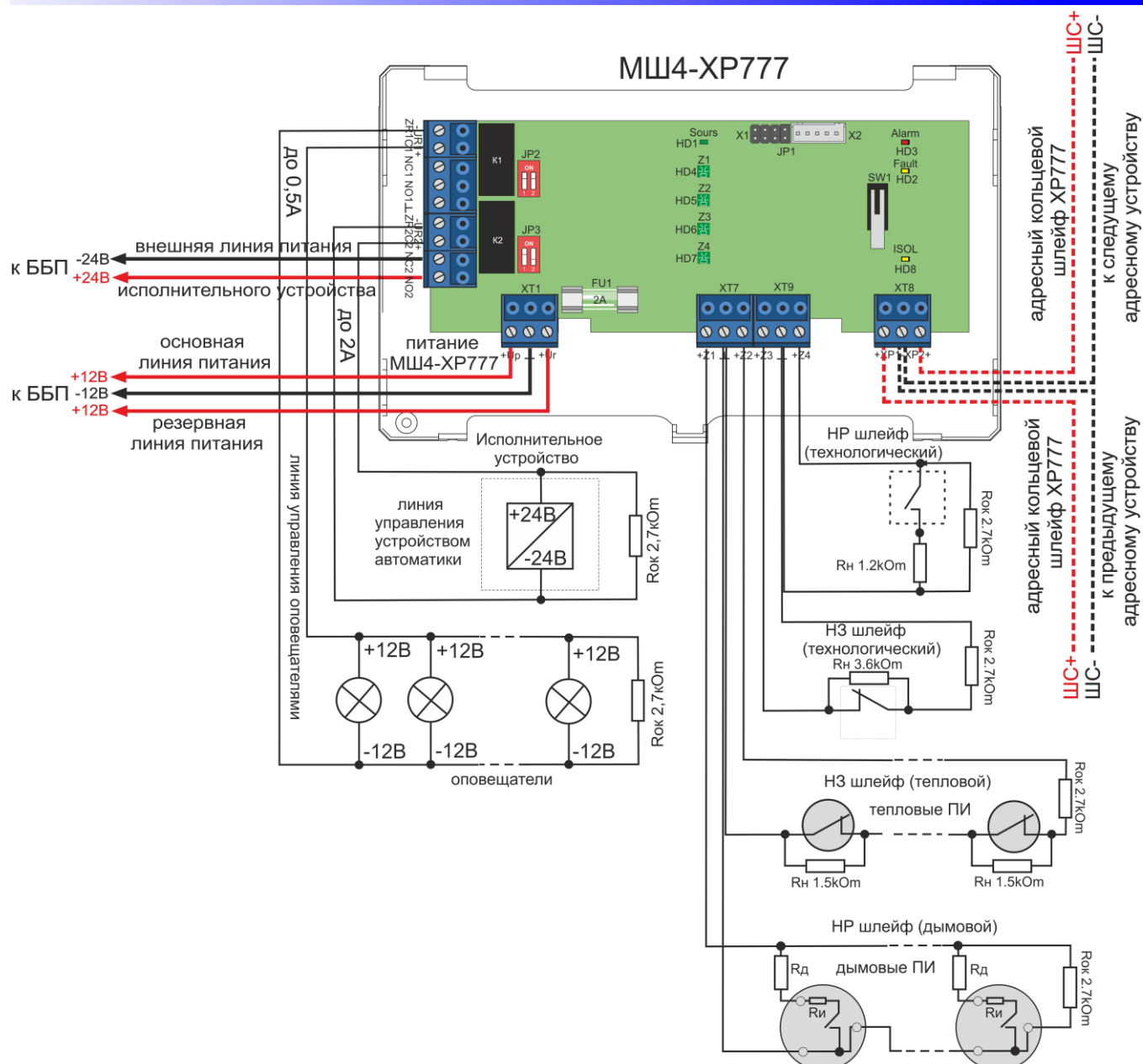
Рисунок 47. Схема подключения МШ4-ХР777
