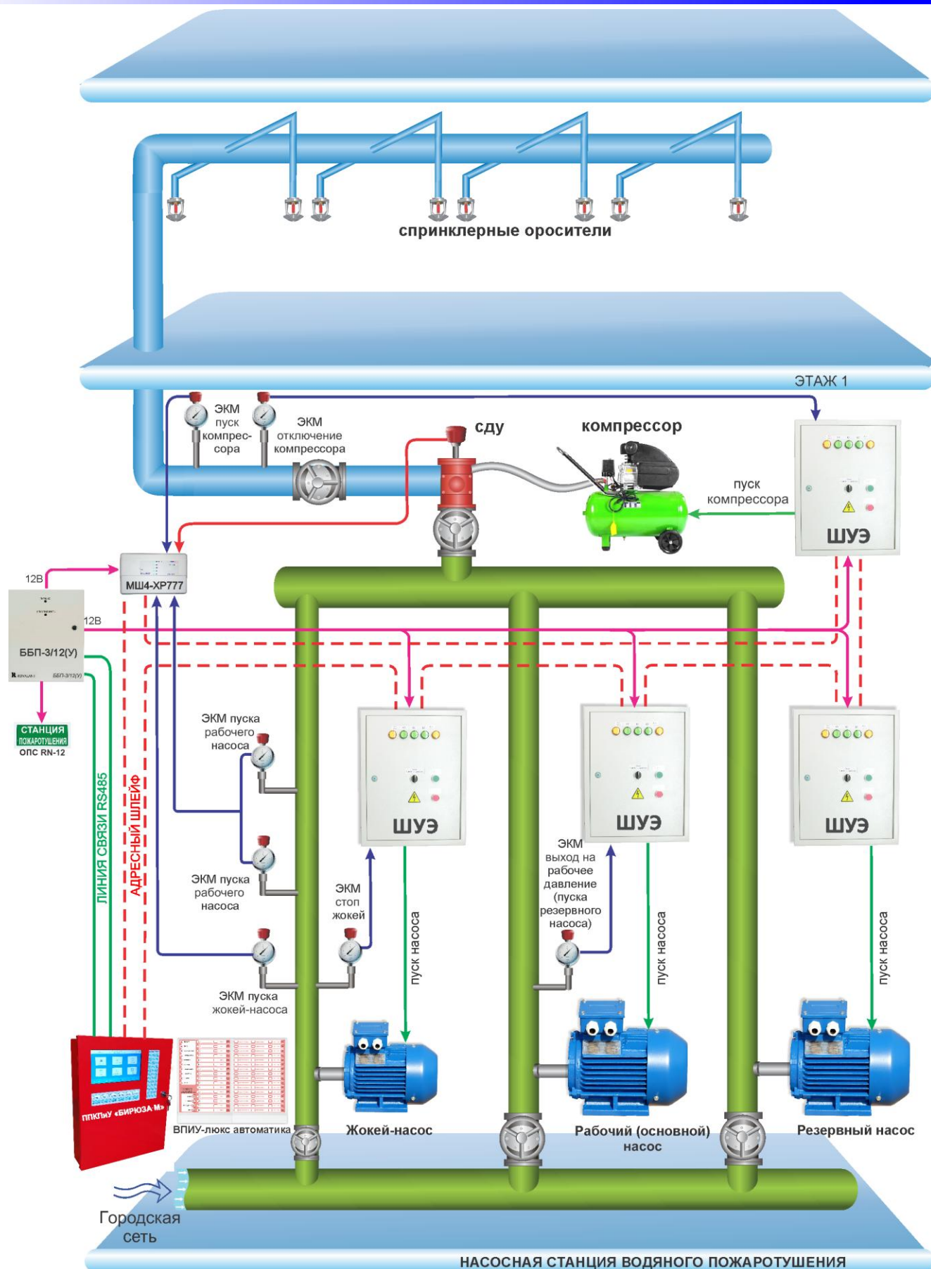
Рисунок 110. Автоматизация спринклерной установки воздухозаполненной системы водяного АПТ.
