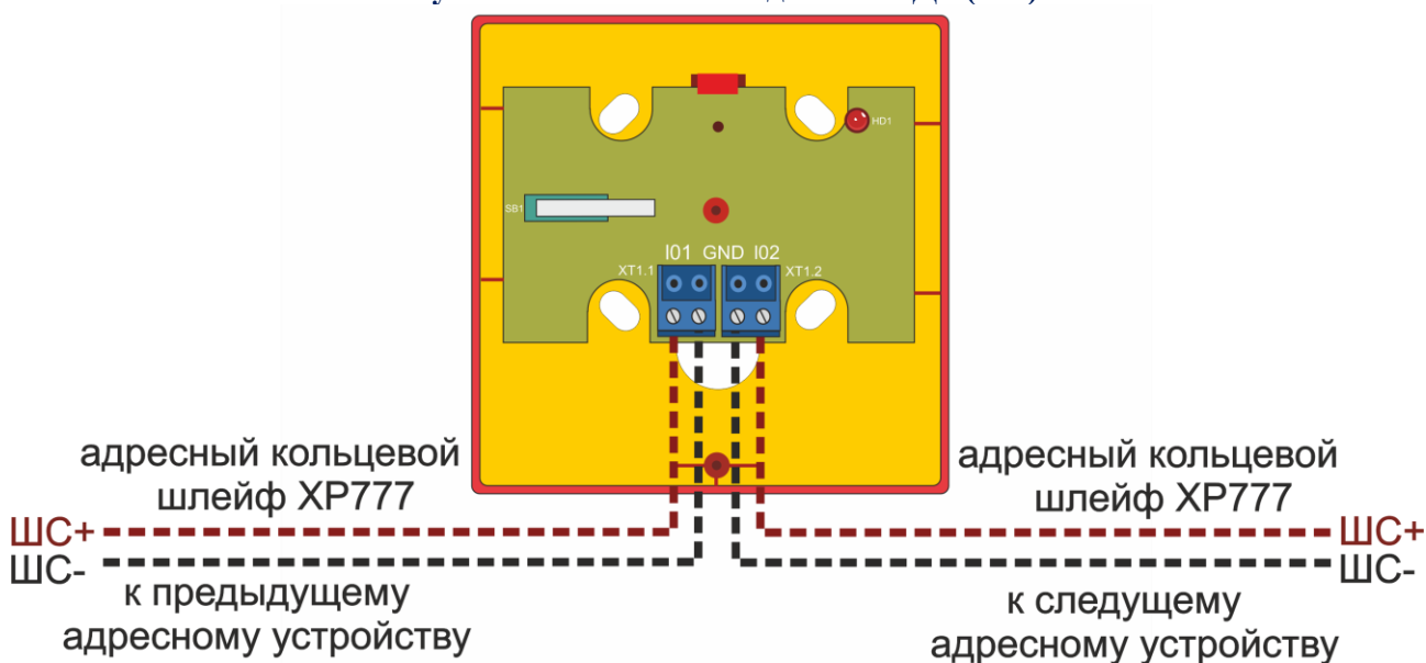
Рисунок 39. Схема подключения RF05-УДП(ДУ) и RF05-УДП(ПТ)
