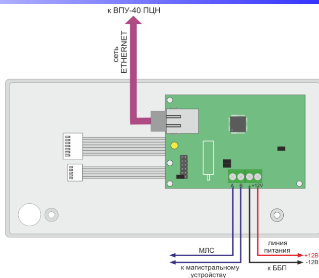
Рисунок 90. Схема подключения ИС-ЕТН/485 для организации связи МУ с ПЦН
