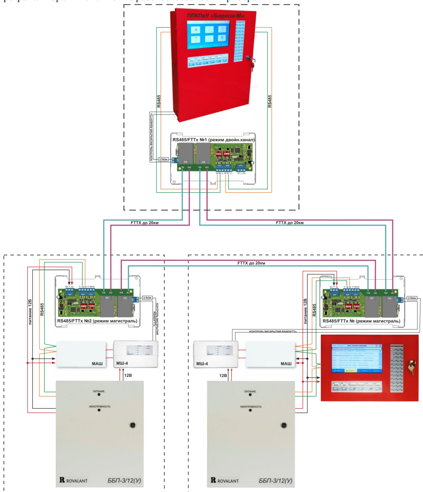
Рисунок 89. Схема организации оптоволоконной линии связи для ППКПиУ «Бирюза-М»
