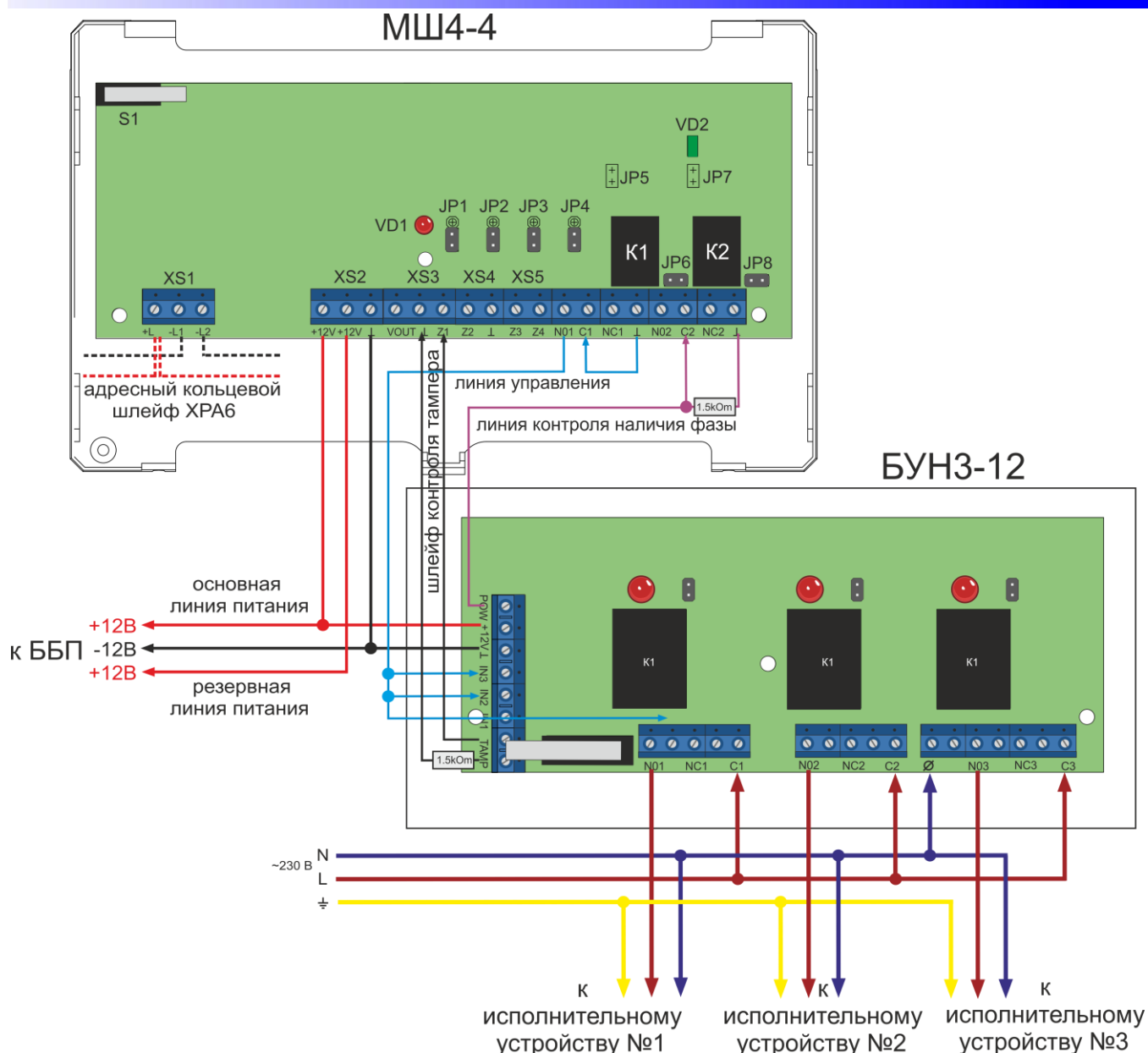
Рисунок 95. Схема подключения БУНЗ-12 к МШ4-4
