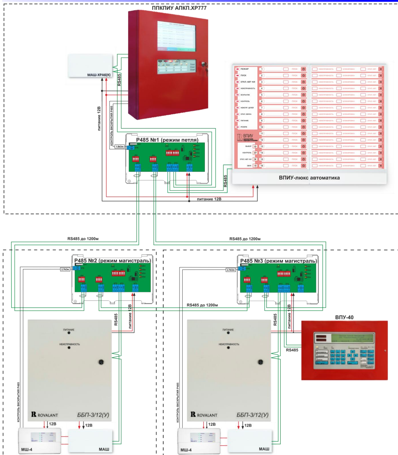
Рисунок 85. Схема организации защищенной ОЛС для ППКПиУ АПКП.XP777
