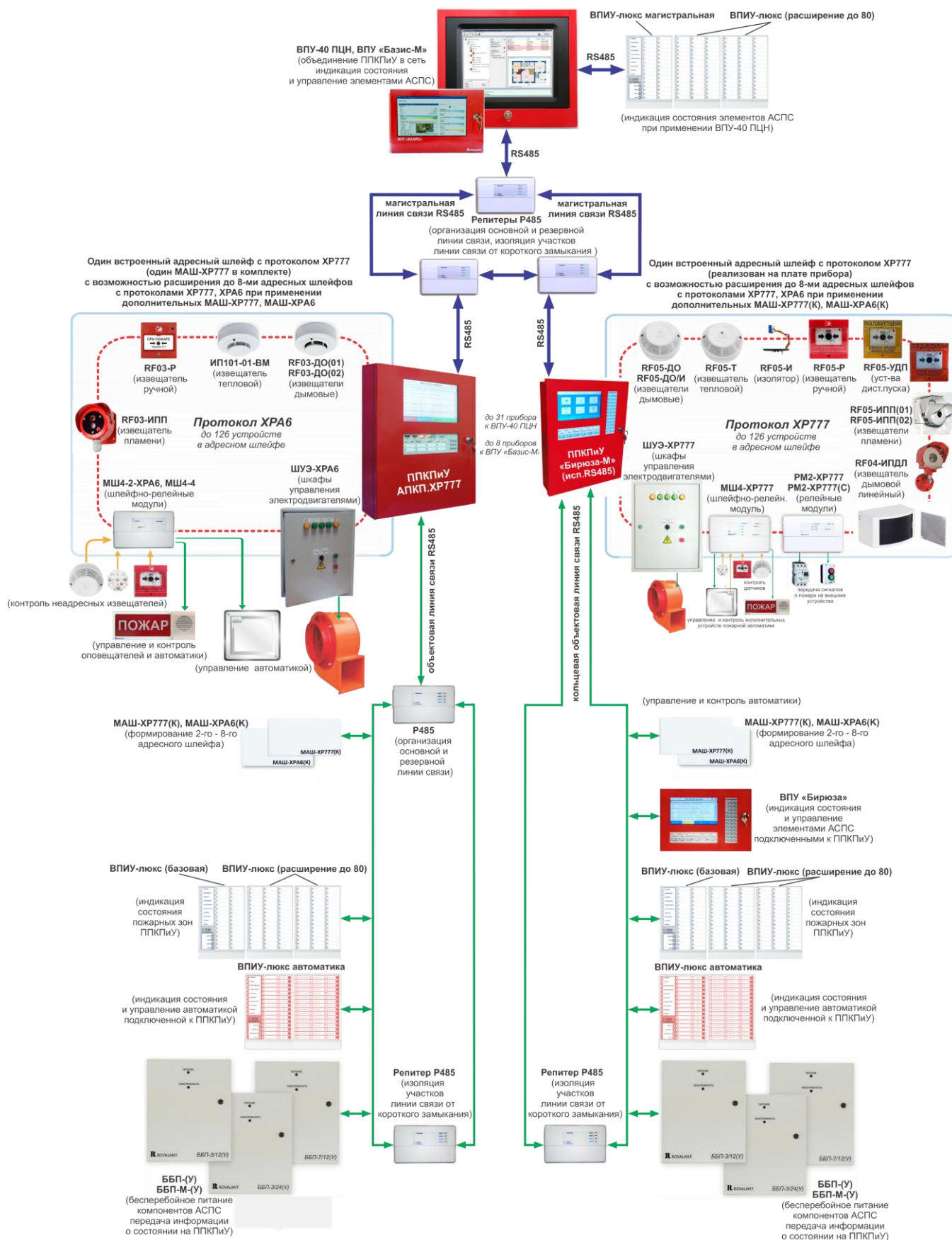
Рисунок 1. Структурная схема АСПС при использовании линии связи стандарта RS485
