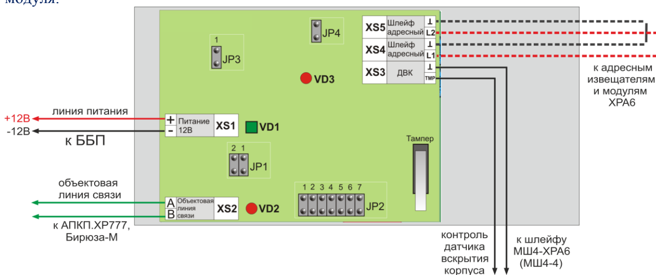
Рисунок 53. Схема подключения МАШ-ХРА6(К)
