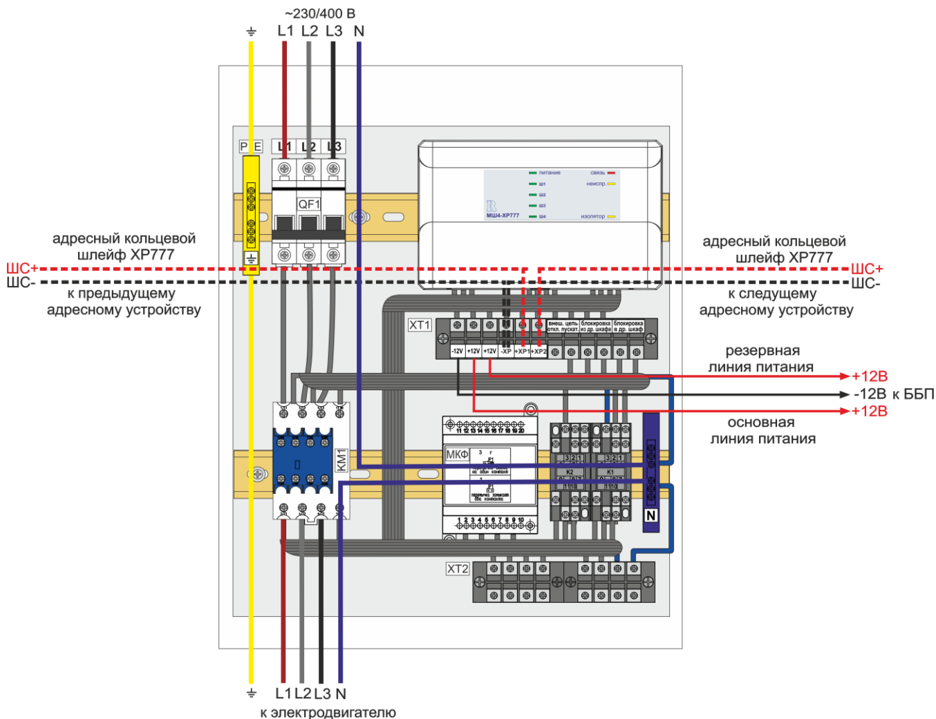
Рисунок 45. Схема подключения ШУЭ-ХР777
