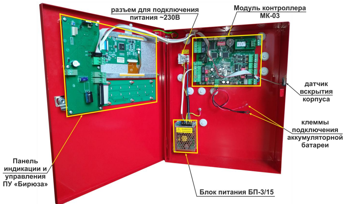
Рисунок 12. Внешний вид ППКПиУ «Бирюза-М» с открытой лицевой панелью
