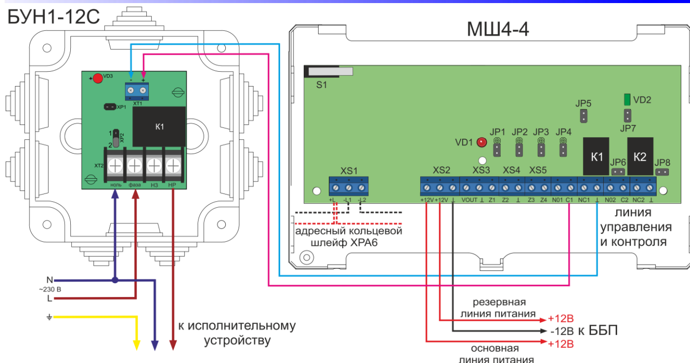
Рисунок 93. Схема подключения БУН1-12С к МШ4-4
