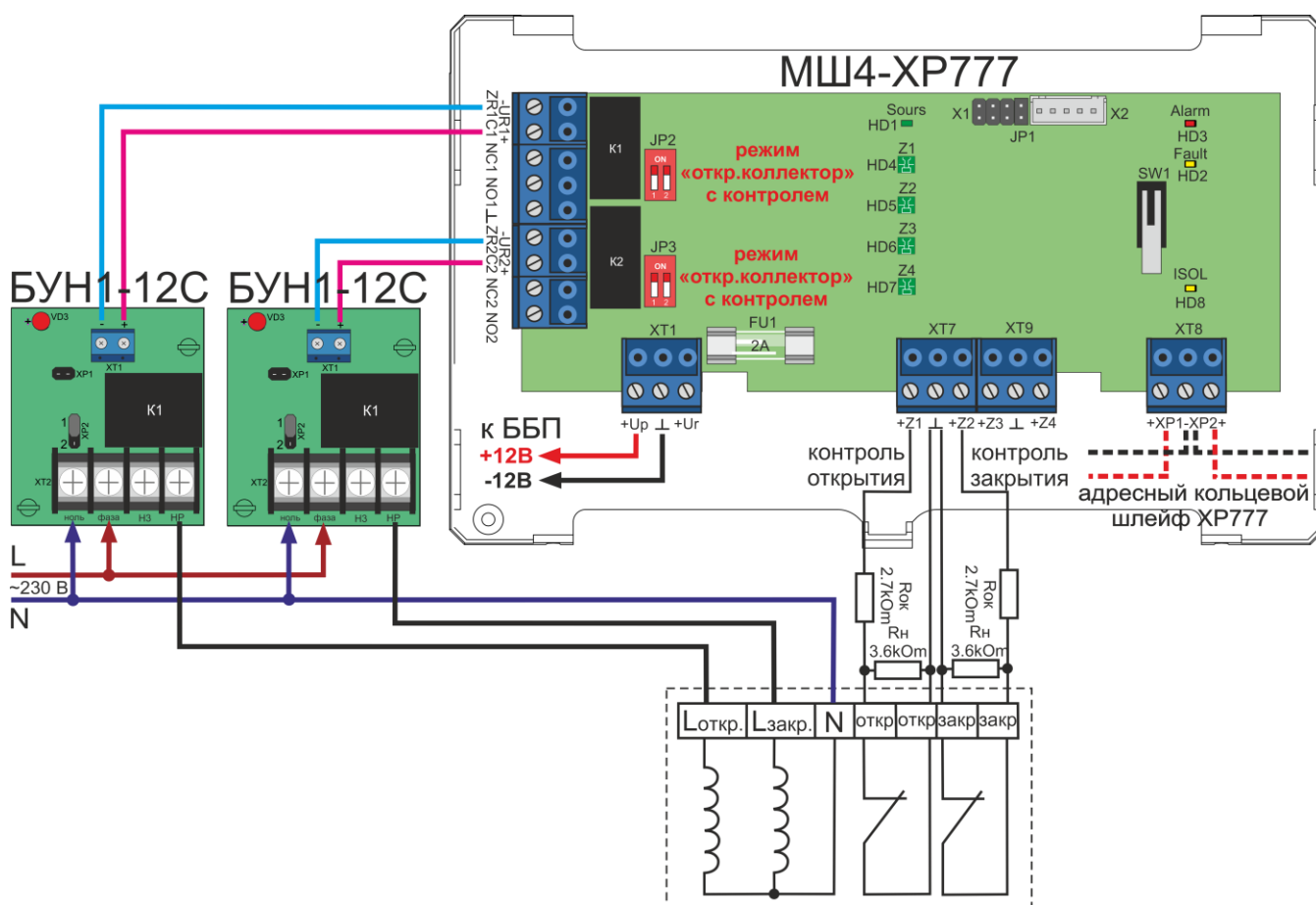
Рисунок 103. Схема подключения реверсивного 3-х проводного привода с напряжением питания 230В
