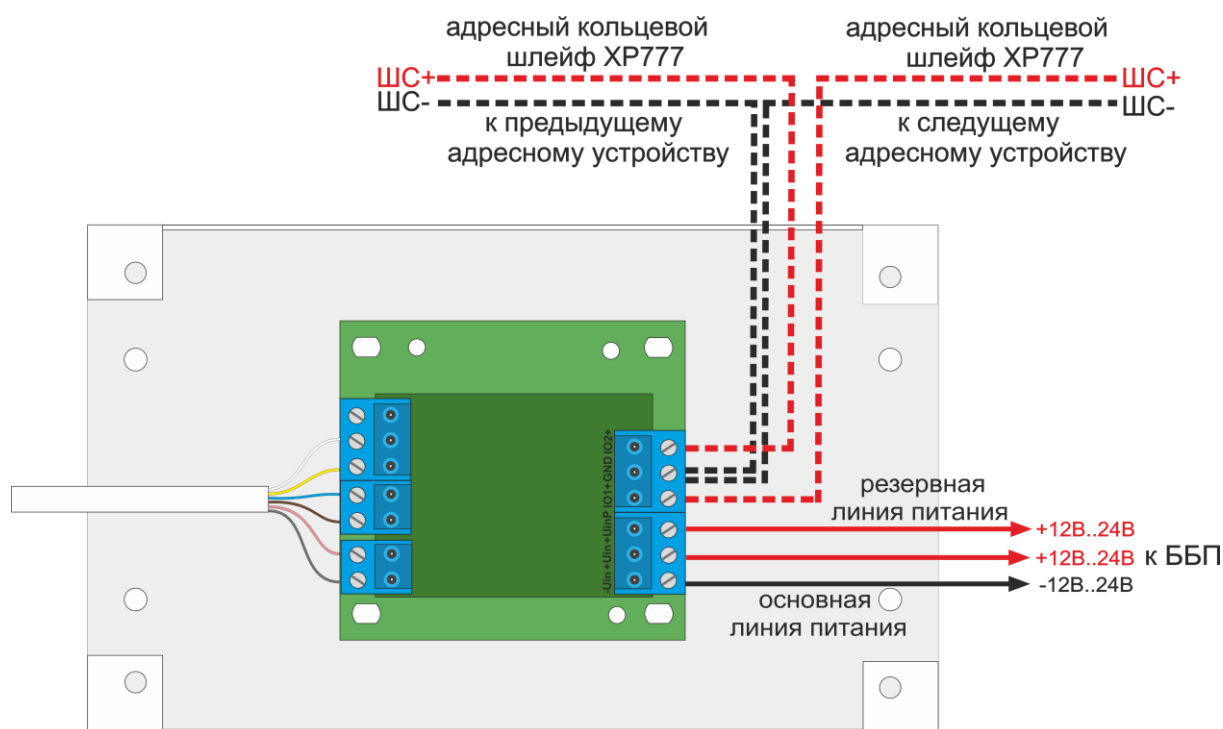
Рисунок 41. Схема подключения RF04-ИПДЛ
