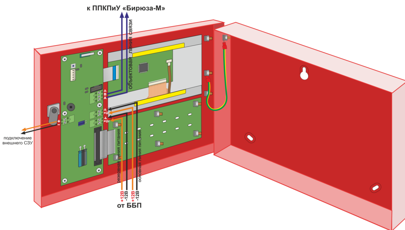
Рисунок 70. Схема подключения ВПУ «Бирюза»
