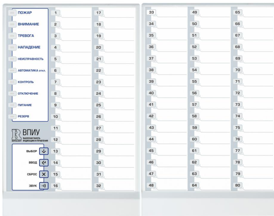
Рисунок 81. Внешний вид ВПИУ-люкс (базовая) с одной ВПИУ-люкс (расширение до 80)
