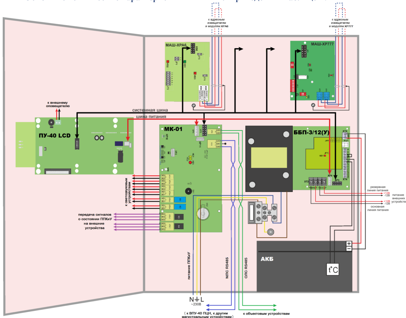
Рисунок 10. Структурная схема внутренних и внешних соединений ППКПиУ АПКП.ХР777
