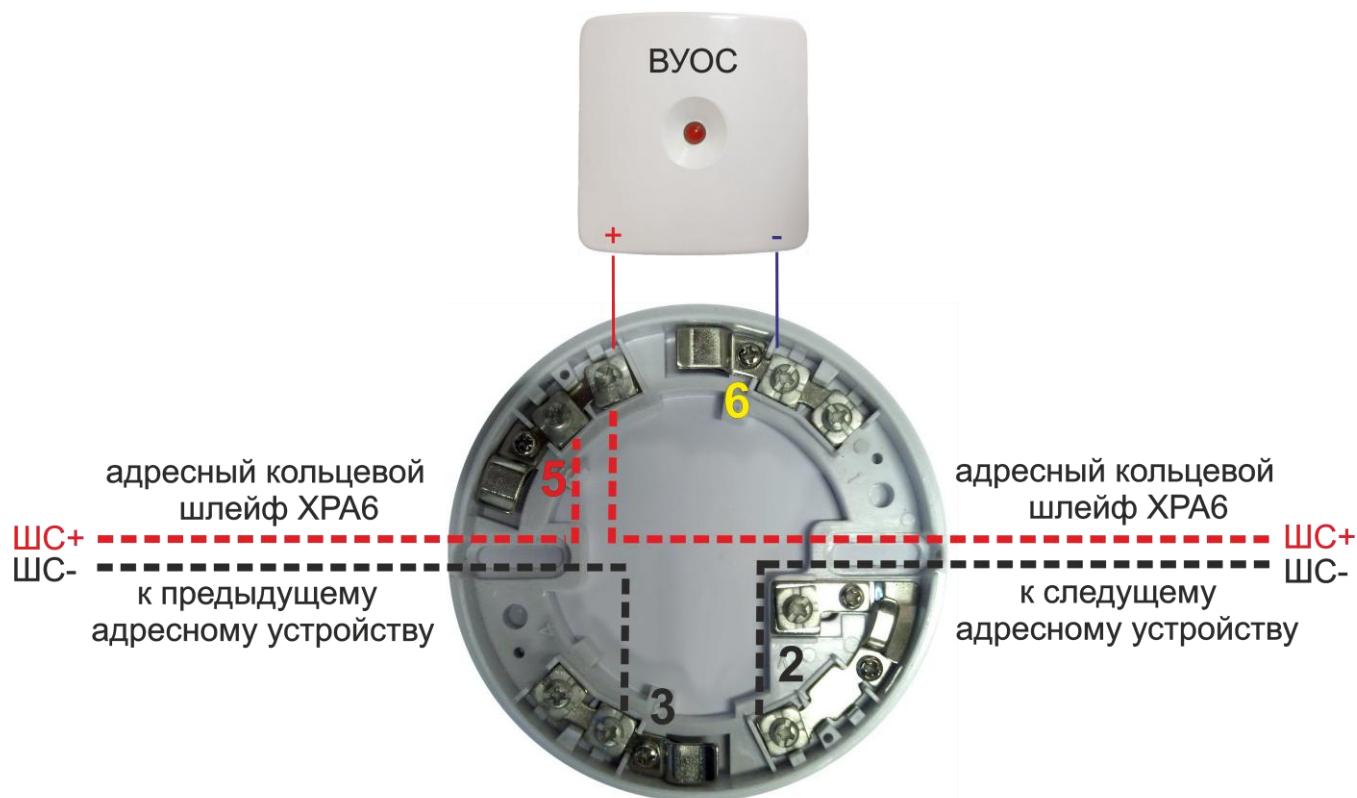
Рисунок 57. Схема подключения ИП101-01-ВМ
