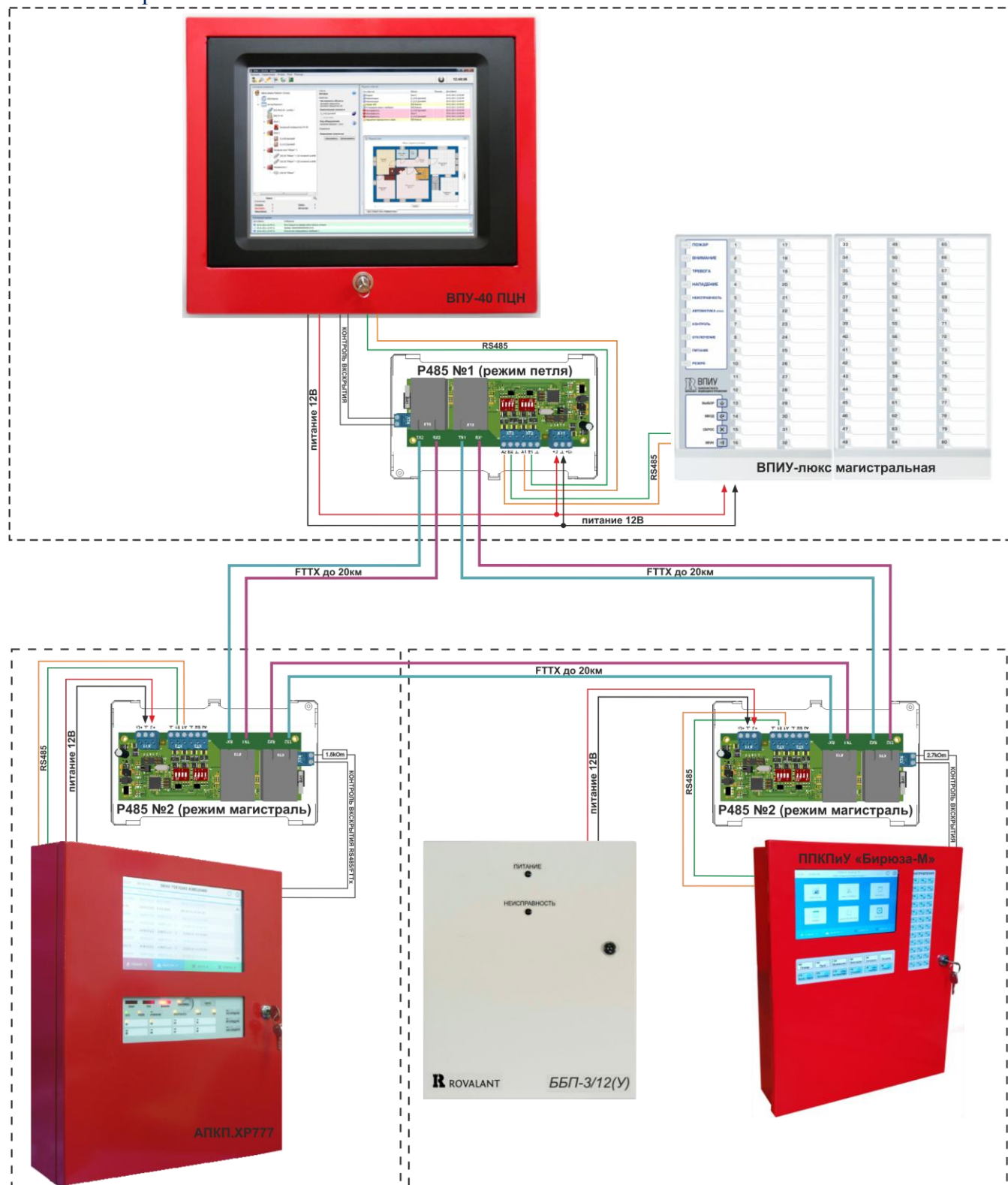
Рисунок 88. Схема организации кольцевой оптоволоконной магистральной линии связи
