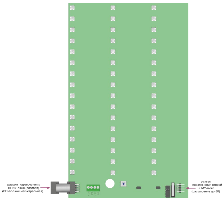
Рисунок 83. Схема подключения ВПИУ-люкс (расширение до 80)
