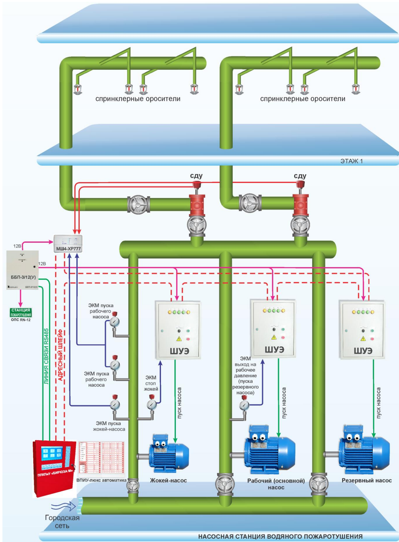
Рисунок 109. Автоматизация спринклерной установки водозаполненной системы водяного АПТ
