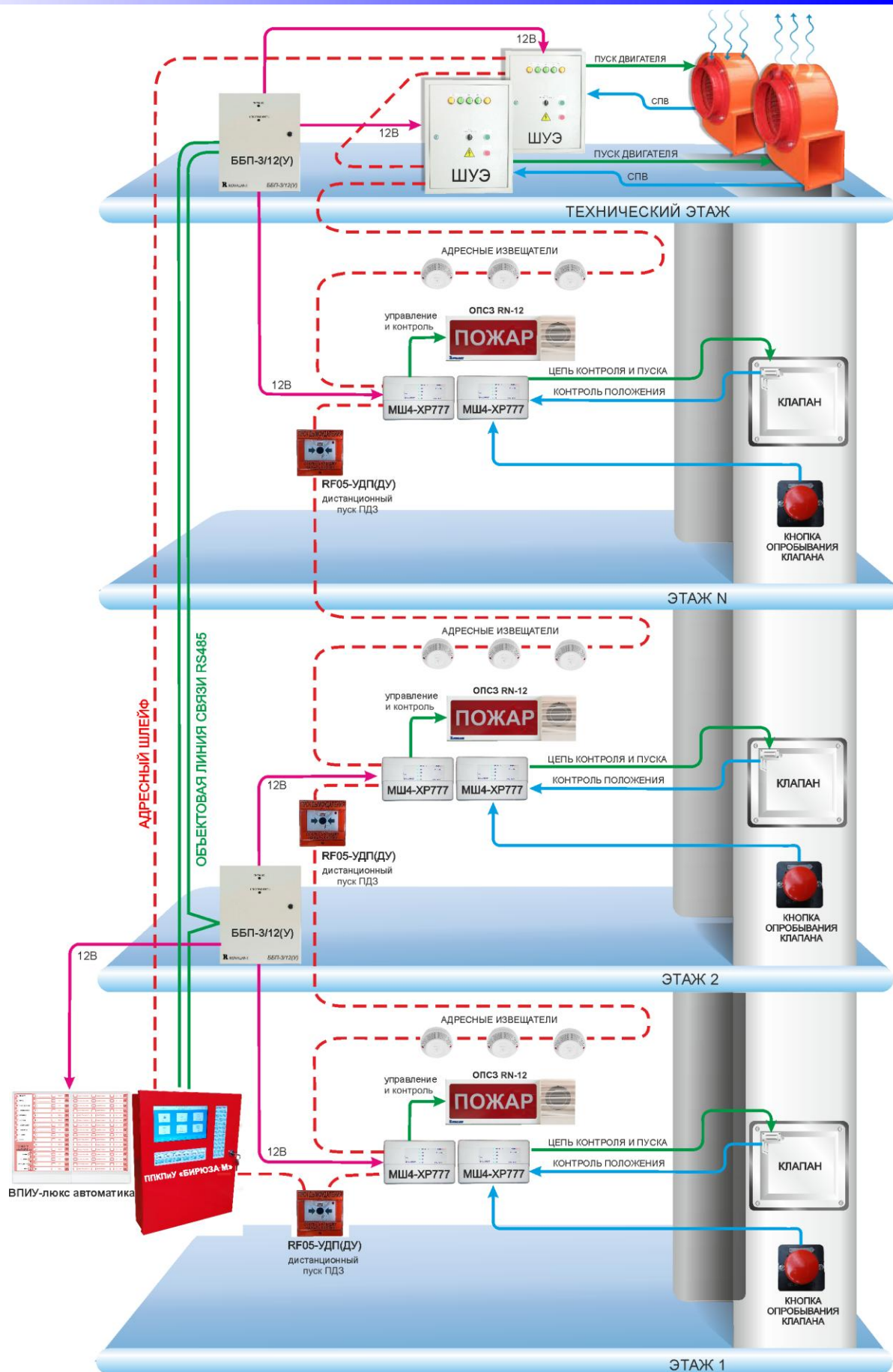
Рисунок 98. Построение системы ПДЗ с использованием адресных извещателей
