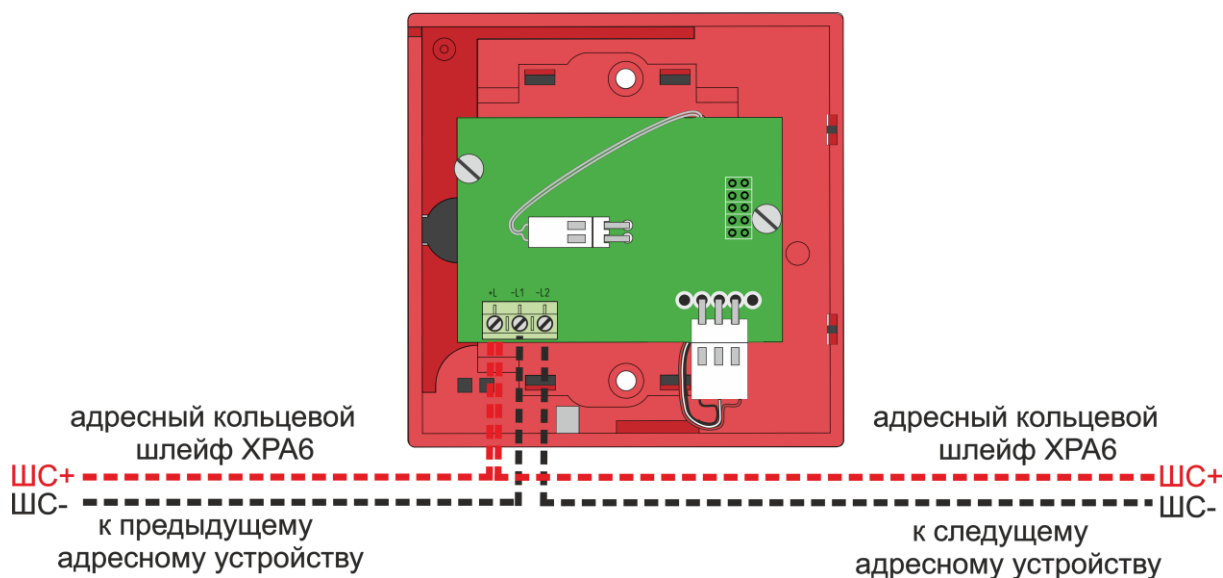
Рисунок 59. Схема подключения RF03-P
