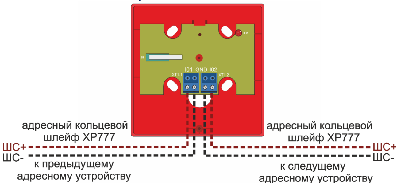
Рисунок 36. Схема подключения RF05-P
