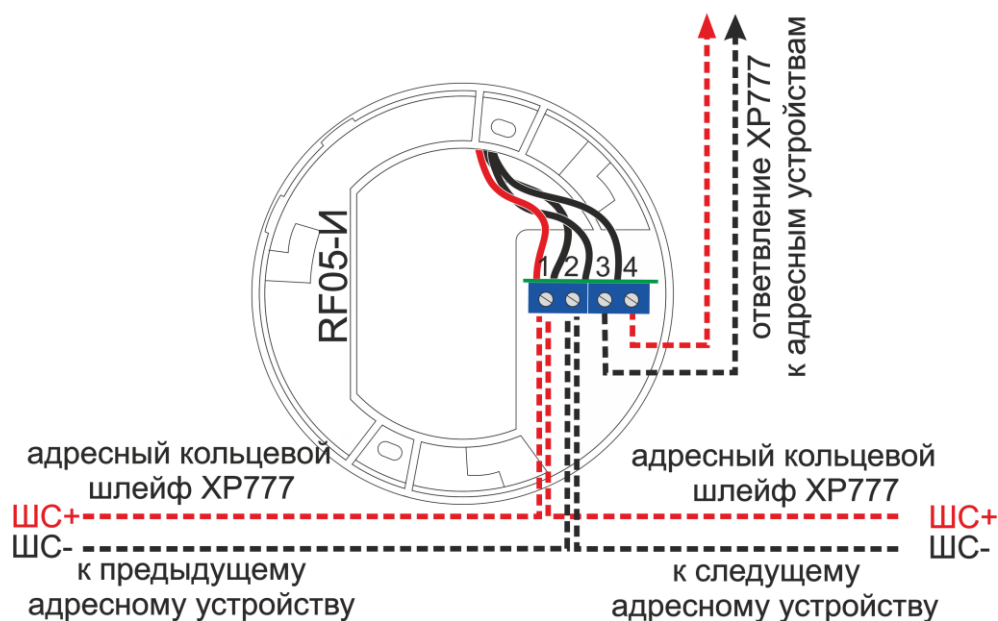
Рисунок 32. Схема подключения RF05-II для построения ответвлений
