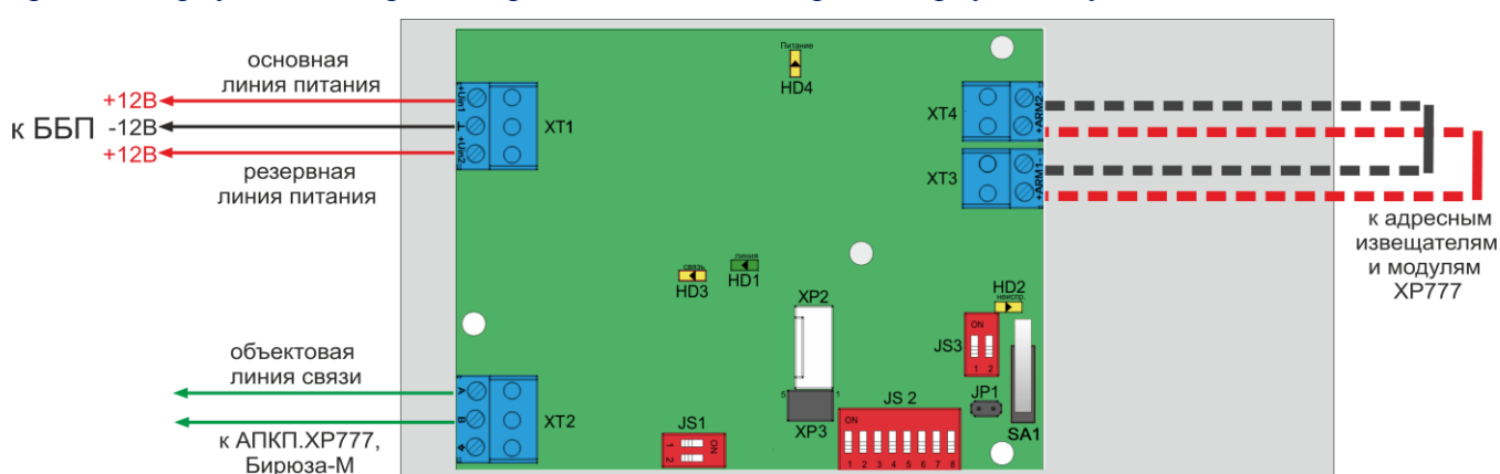
Рисунок 19. Схема подключения МАШ-ХР777(К)
