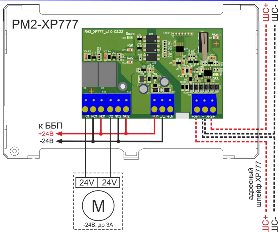
Рисунок 104. Схема управления 2-х проводным реверсивным приводом с напряжением питания 24В
