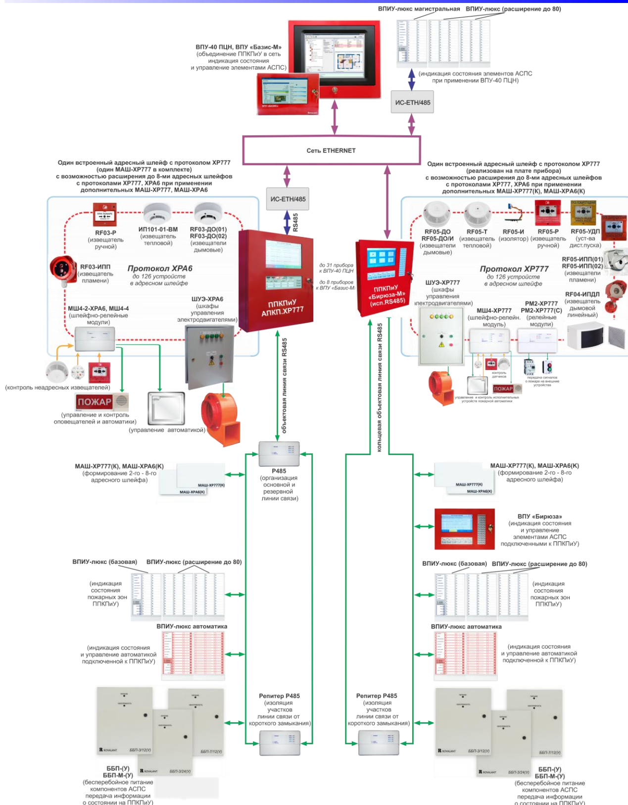
Рисунок 3. Структурная схема АСПС при объединении ППКПиУ по сети ETHERNET
