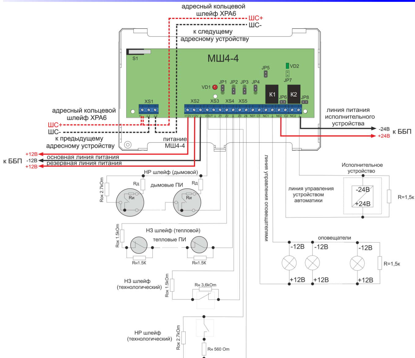
Рисунок 64. Схема подключения МШ4-4
