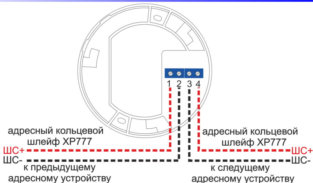
Рисунок 23. Схема подключения RF05-ДО
