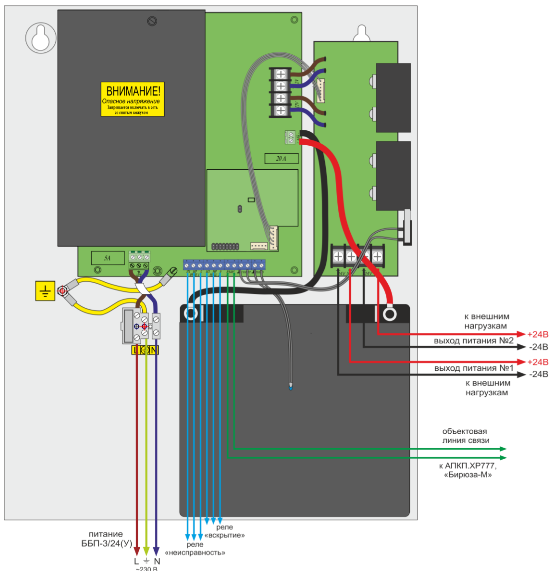
Рисунок 76. Схема подключения ББП-3/24(У)
