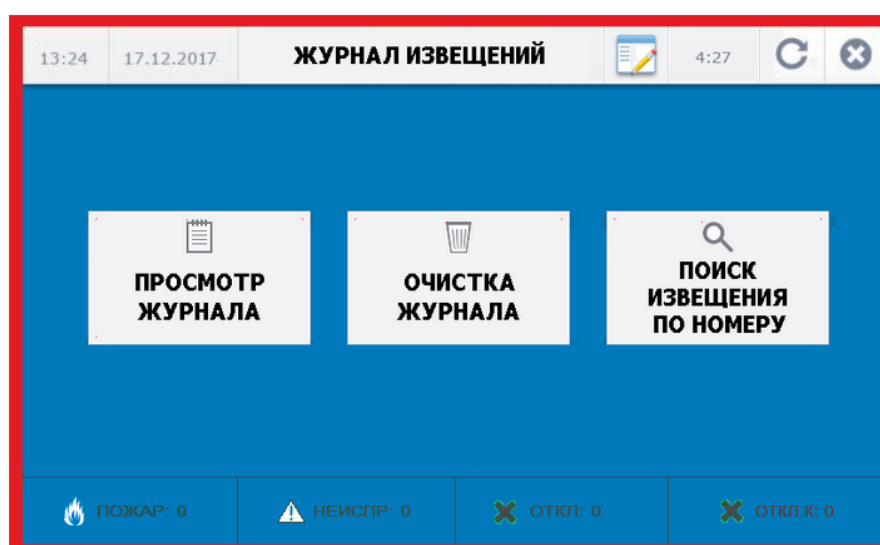
Рисунок 34. Меню «Журнал».
