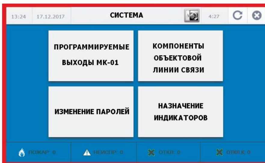
Рисунок 19. Меню «Система».
