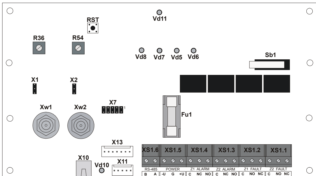
Рисунок 6. Плата управления извещателя «Рубикон-1».
