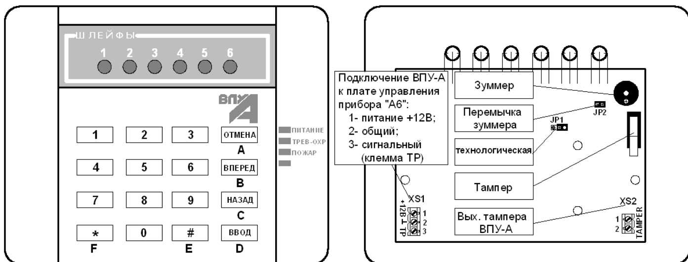
Рисунок 7 – Внешний вид светодиодной клавиатуры ВПУ-А
