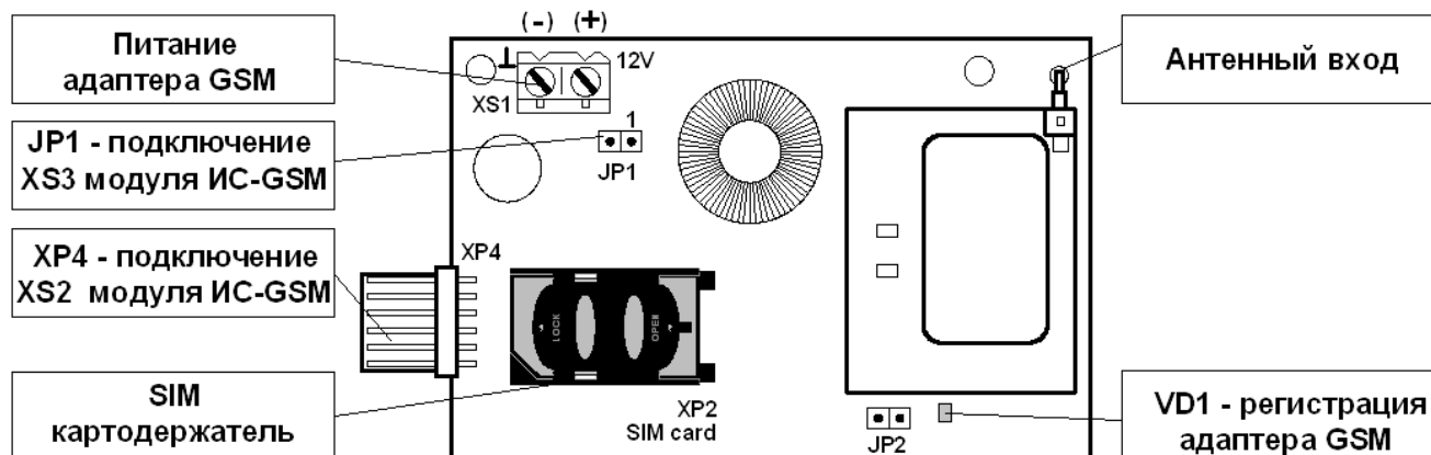
Рисунок 26 - Внешний вид адаптера GSM
