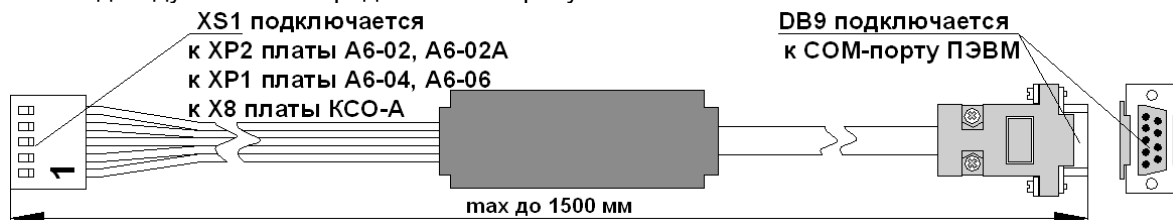
Рисунок 18 – Внешний вид модуля согласования ИС-232
