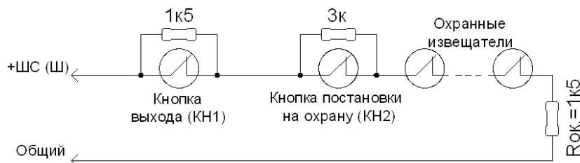
Рисунок 31 – Подключение в шлейф «Кнопки постановки на охрану» и «Кнопки выхода»
