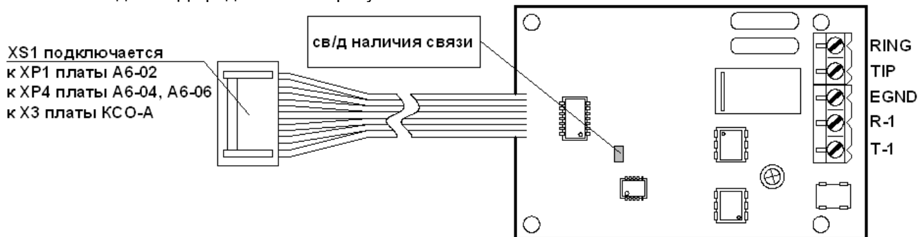
Рисунок 25 – Внешний вид модуля согласования ИС-АД
