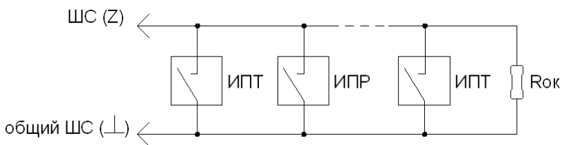
Рисунок 4 - Схема подключения пожарных извещателей с нормально разомкнутыми контактами в пожарный ШС с выдачей сигнала «Пожар» при коротком замыкании ШС
