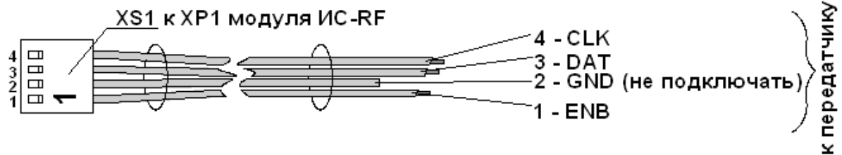
Рисунок 4 – Внешний вид шлейфа-адаптера при работе прибора «А6» в составе РСПИ «Андромеда» («PIMA»)
