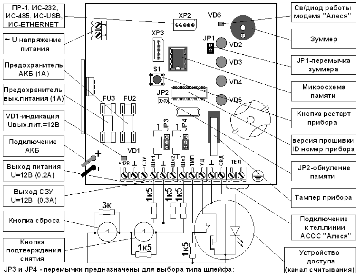
Рисунок 1 – Внешний вид платы управления прибора «А6» исполнения А6-02
