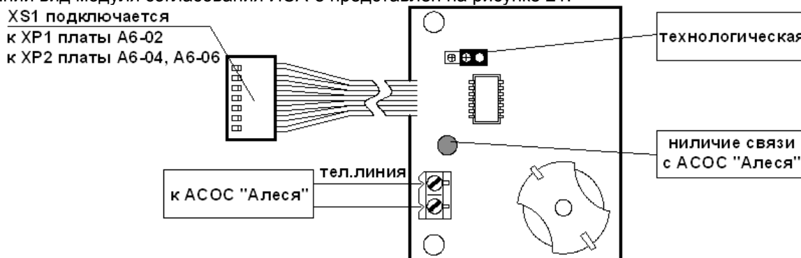
Рисунок 21 – Внешний вид модуля согласования ИСА-8
