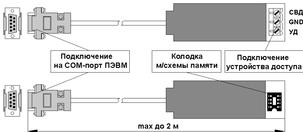
Рисунок 29 – Внешний вид программатора PROG-1 с возможностью подключения к COM-порту ПЭВМ
