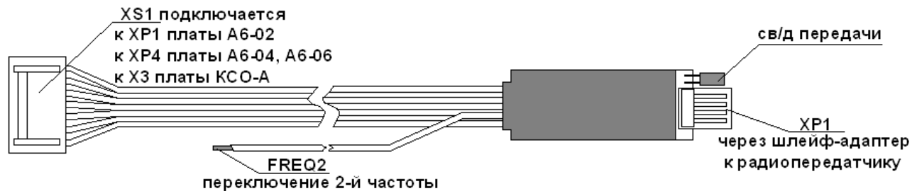
Рисунок 23 – Внешний вид модуля согласования ИС-RF при работе в составе РСПИ «Андромеда» («PIMA»)
