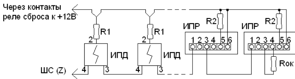
Рисунок 12 - Схема подключения ручных извещателей ИПР-Ксу в пожарный ШС совместно с дымовыми 2-х проводными извещателями ИП212 моделей 5М, 44, 54Т, 3СУ, 41М. Перемычки ИПР: J1 установлена, J2 и J3 сняты
