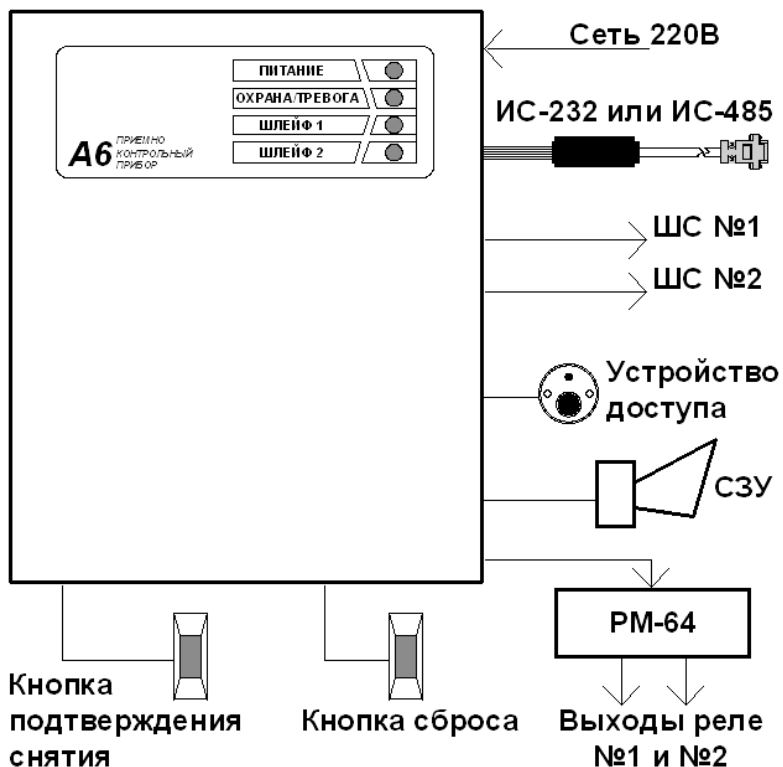
Рисунок 1 – Внешний вид прибора «А6» (исполнение А6-02)
