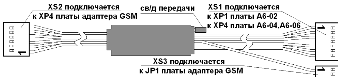
Рисунок 25 - Внешний вид модуля согласования ИС-GSM
