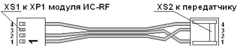
Рисунок 1 – Внешний вид шлейфа-адаптера при работе прибора «А6» в составе РСПИ «МАЯК» («STARS»), «RRT Laboratorija»
