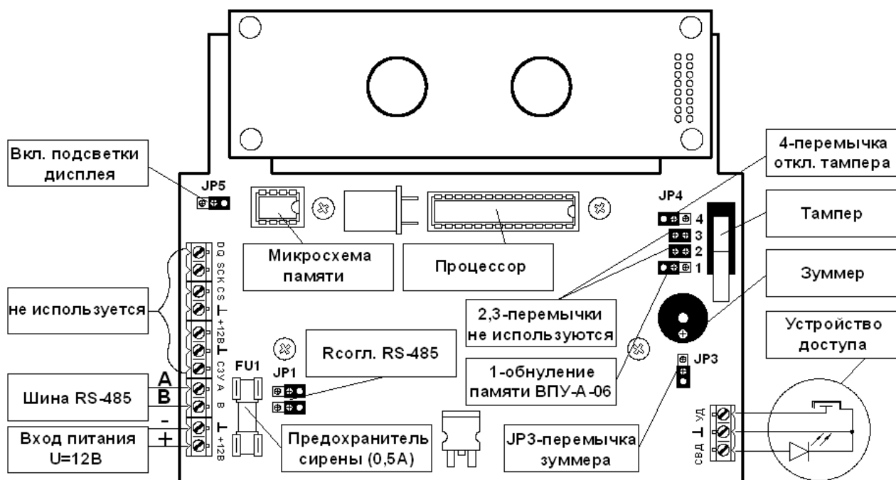
Рисунок 10 - Внешний вид клавиатуры ВПУ-А-06 со снятой задней крышкой
