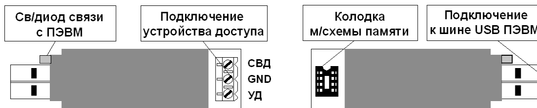
Рисунок 28 – Внешний вид программатора PROG-1 с возможностью подключения к шине USB ПЭВМ
