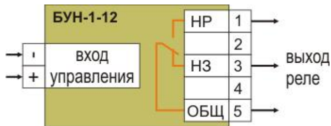
Рисунок 1. Подключение БУН 1-12.
