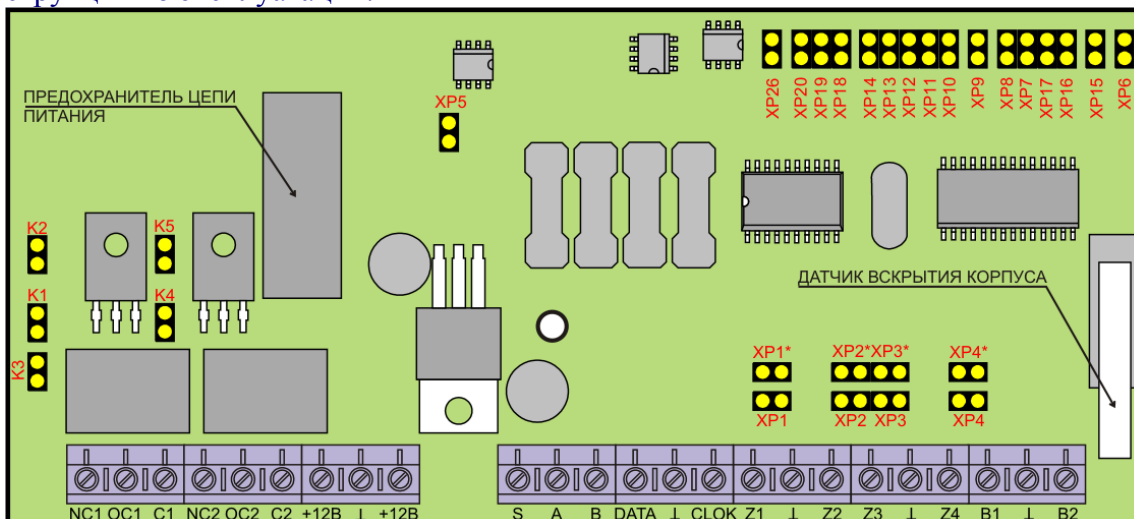
Рисунок 1. Внешний вид платы АБ4.
