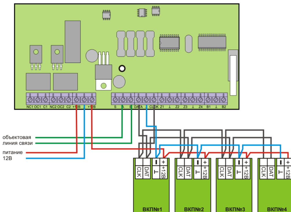
Рисунок 11. Типовая схема подключения ВКП к АБ4.
